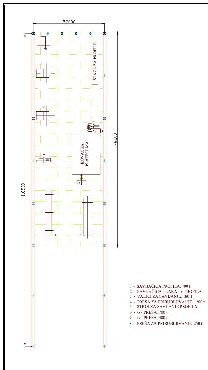
Slika 33. Novi raspored strojeva za oblikovanje limova i profila
