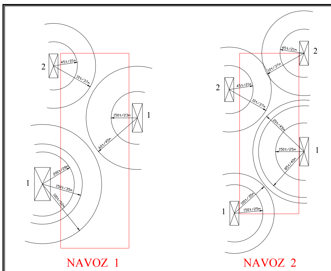
Slika 28. Dizalice uz navoze
