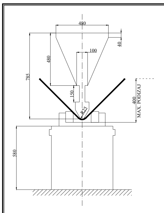
Slika 23. Poprečni presjek velike preše za savijanje limova
