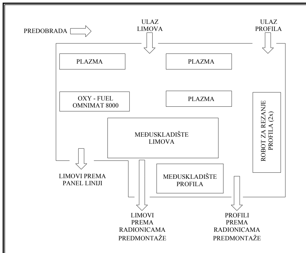
Slika 14. Shema radionice obrade
