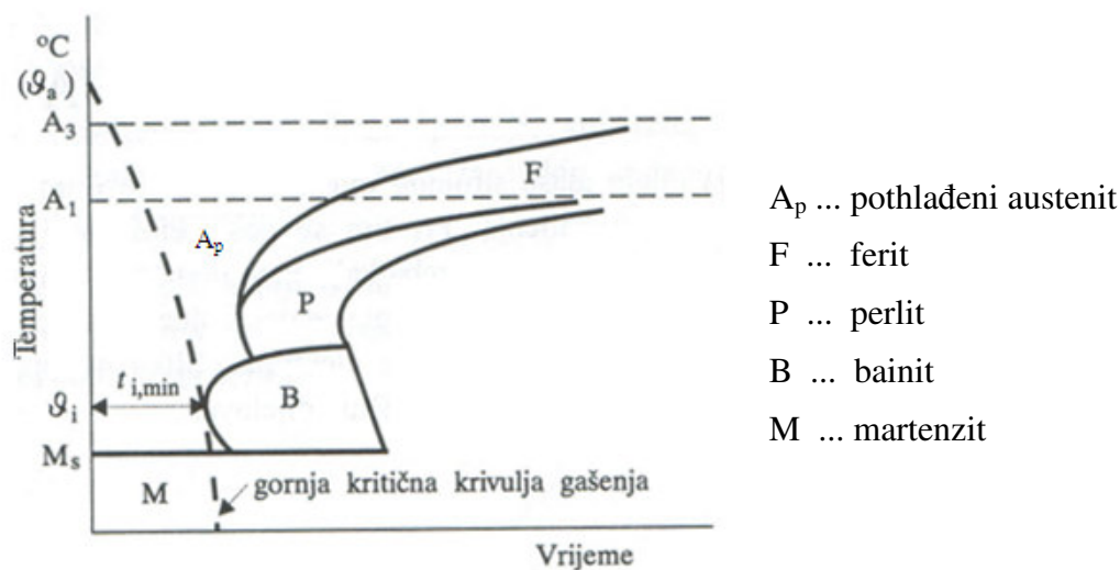
Slika 4. Shematski prikaz određivanja gornje kritične brzine gašenja (na primjeru kaljenja čelika s manje od 0,8%C) [1]
