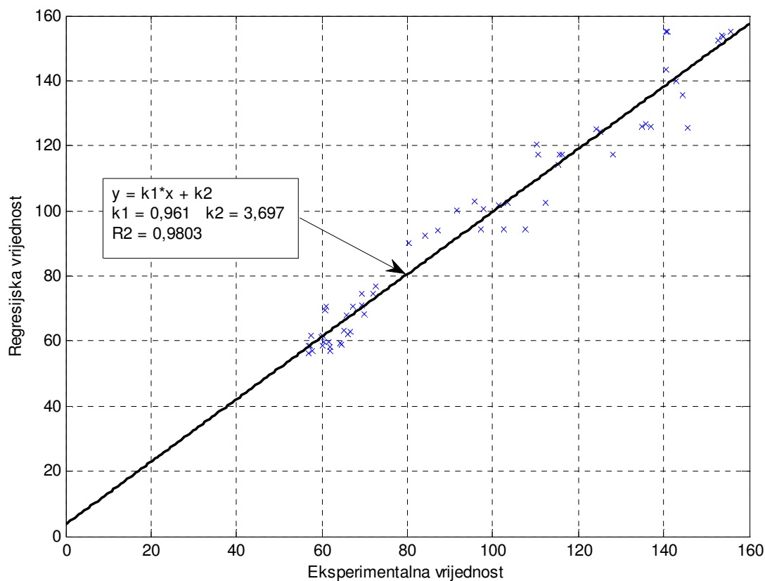
Slika 42: Maksimalna brzina gašenja – usporedba eksperimentalnih i modelom dobivenih vrijednosti tehnoloških svojstava
