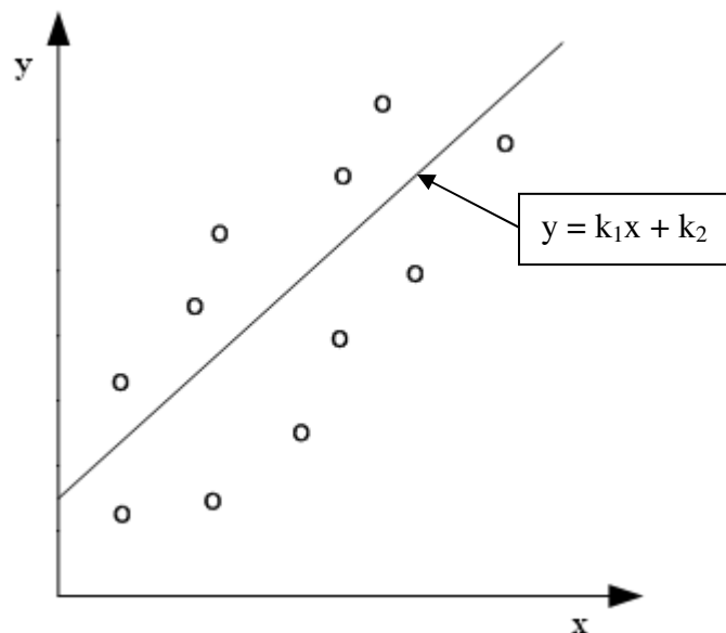
Slika 9: Linearna regresija
