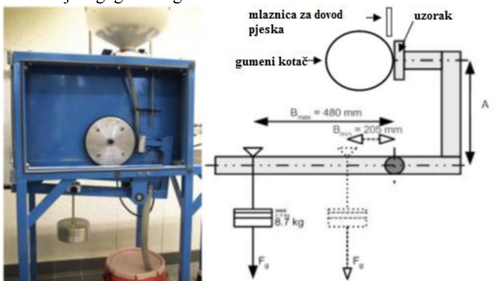
Slika 20. Uređaj za ispitivanje otpornosti na abrazijsko trošenje [8]
