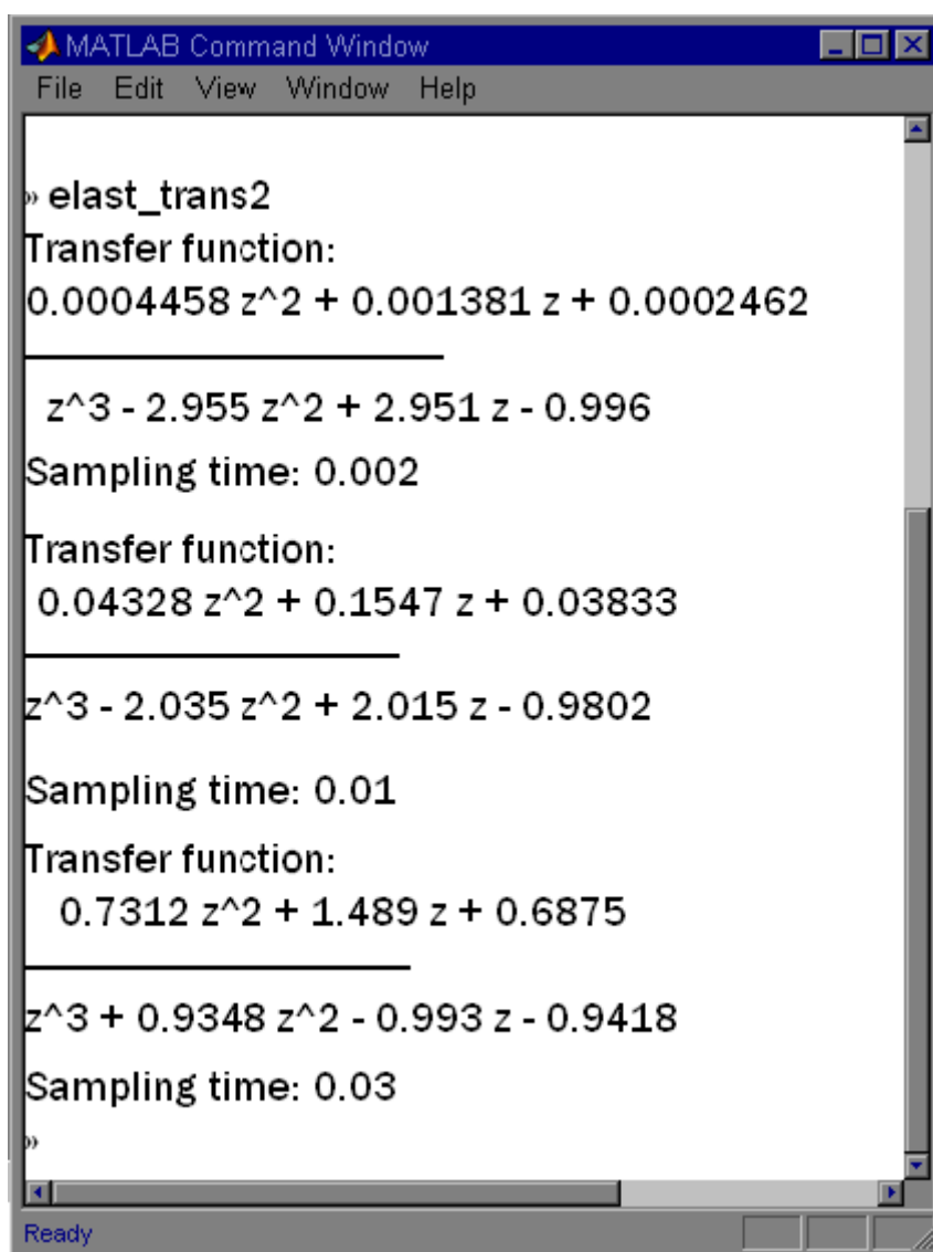
Slika 6. Prijenosne funkcije (vježbe iz ndu)
