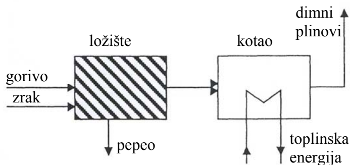
Slika 6. Proces izgaranja [5]
