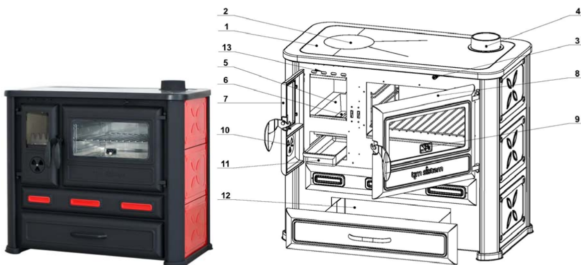
Slika 11. Vanjski izgled i dijelovi tipičnog štednjaka [11]
