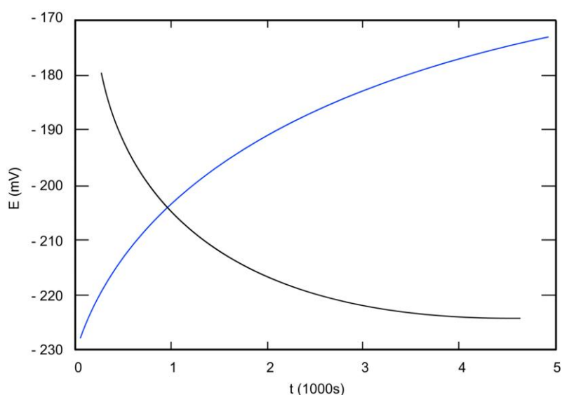
Slika 20. Određivanje potencijala otvorenog strujnog kruga E_{ok} [23]
