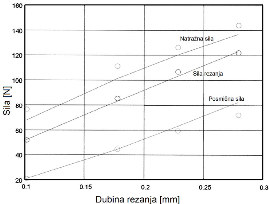
Slika 3.1.1. Promjena iznosa sila s obziroma na posmak kod nepotrošenog alata [11].
