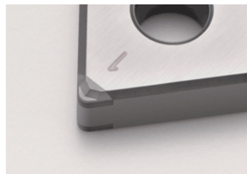
Slika 3.3.5.2. Najnoviji CBN alat tvrtke sumitomo s integriranim lomačem čestice. Prvi proizvedeni te vrste. Služi za tvrdo-meko tokarenje tvrtke sumitomo [19].
