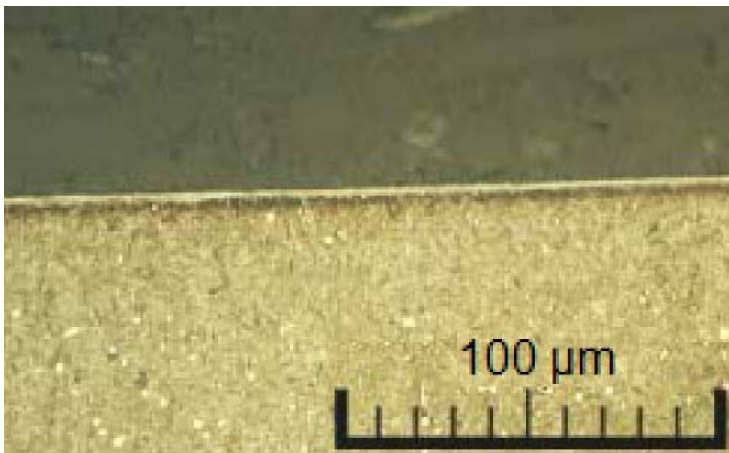
Slika 3.3.1.2. Mikrostruktura kaljenog čelika nakon procesa tvrdog suhog tokarenja [15].
