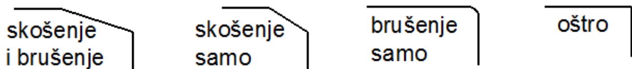
Slika 3.3.1.1. Vrsta pripremljenih oštrica za CBN reznih oštrica [10].
