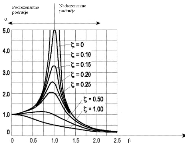
Slika 2. Faktor dinamičnosti \alpha(\beta)
