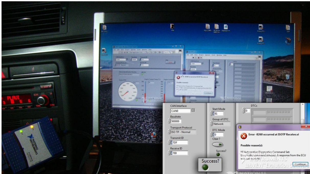
Slika 5.21. Programsko sučelje za očitavanje DTC-ova na vozilu Audi A4.
