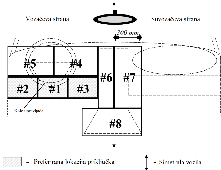
Slika 2.6. Dozvoljena mjesta pozicije dijagnostičkog priključka [5]
