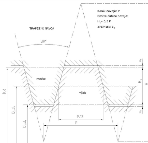
Slika 11. Dimenzije trapeznog navoja
