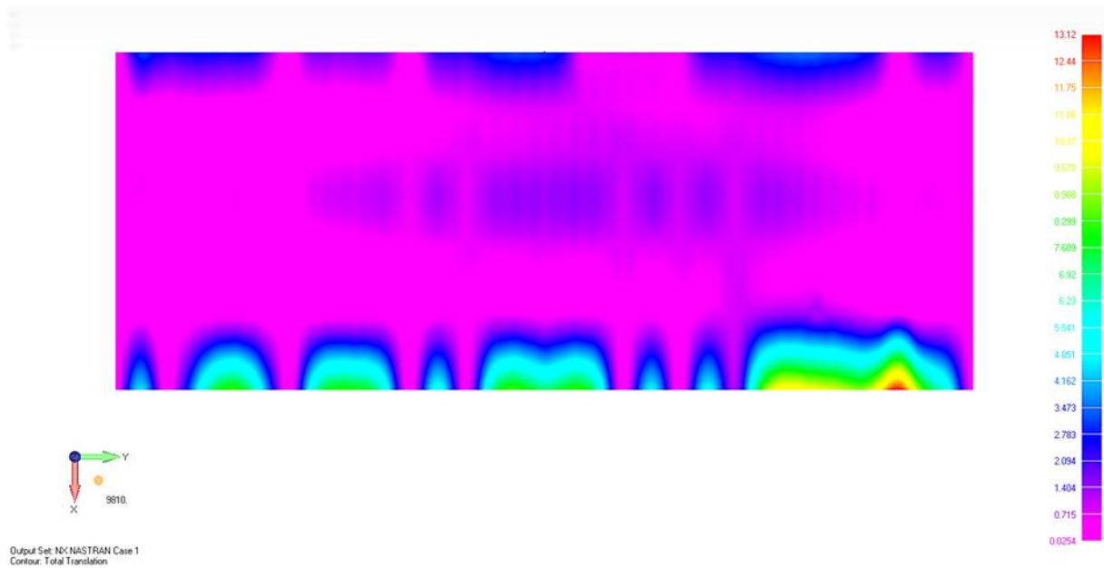
Slika 67. Deformacije na palubi 8 sa uporama, bez kabina
