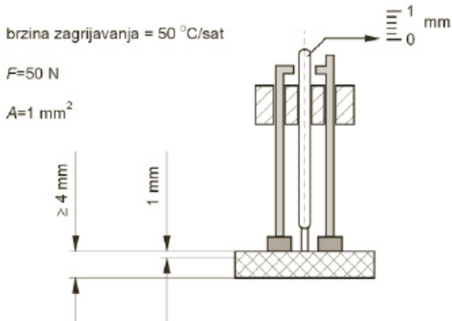
Slika 20. Određivanje temperature omekšavanja po VICAT-u.
