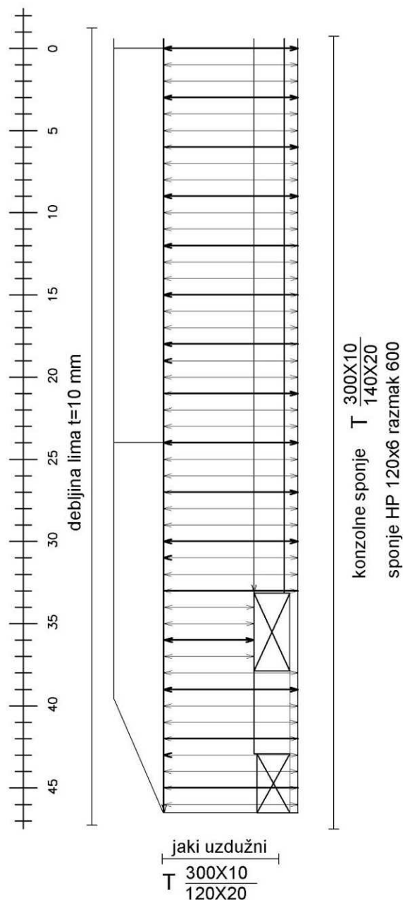
Slika 22: Konstrukcija međupalube
