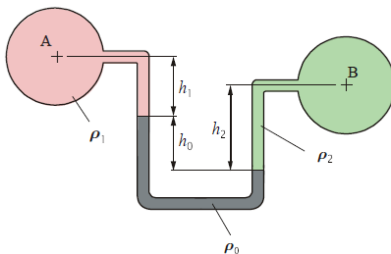
Slika 2-2 Diferencijalni manometar [6]
