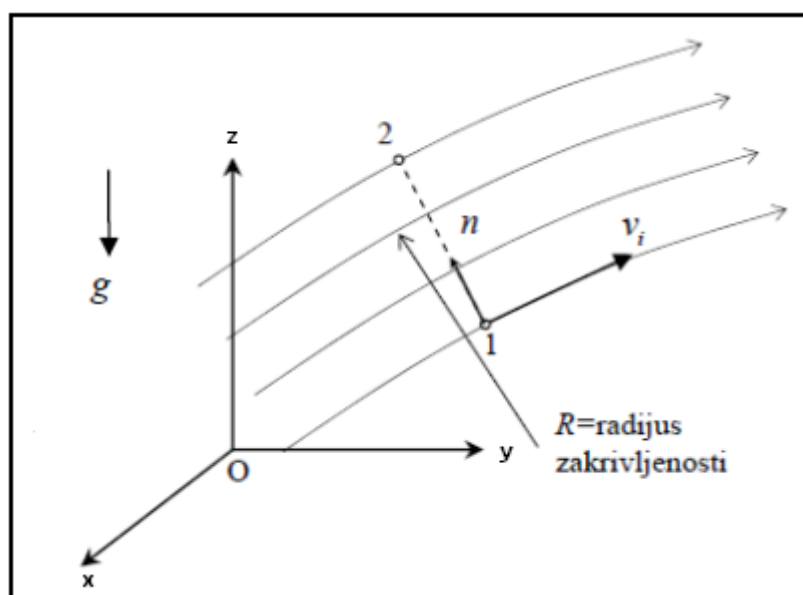
Slika 2-1 Promjena tlaka okomito na strujnice [6]
