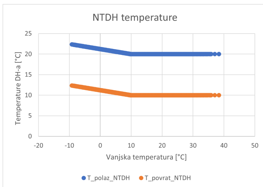
Slika 19 NTDH temperature u ovisnosti o okolišu
