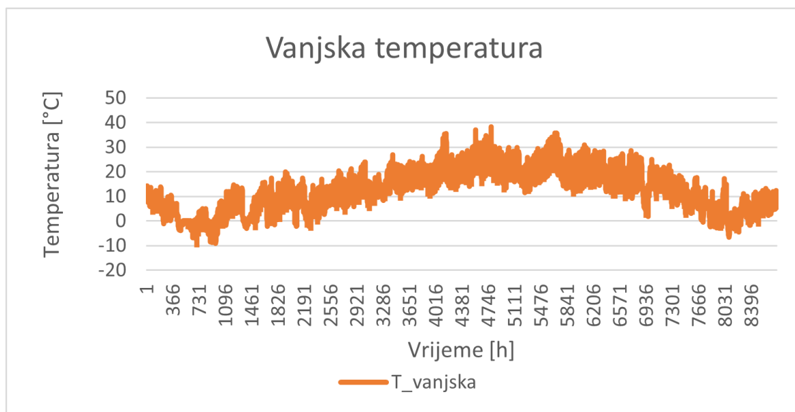
Slika 18 Kretanje vanjske temperature grada Karlovca unutar godine
