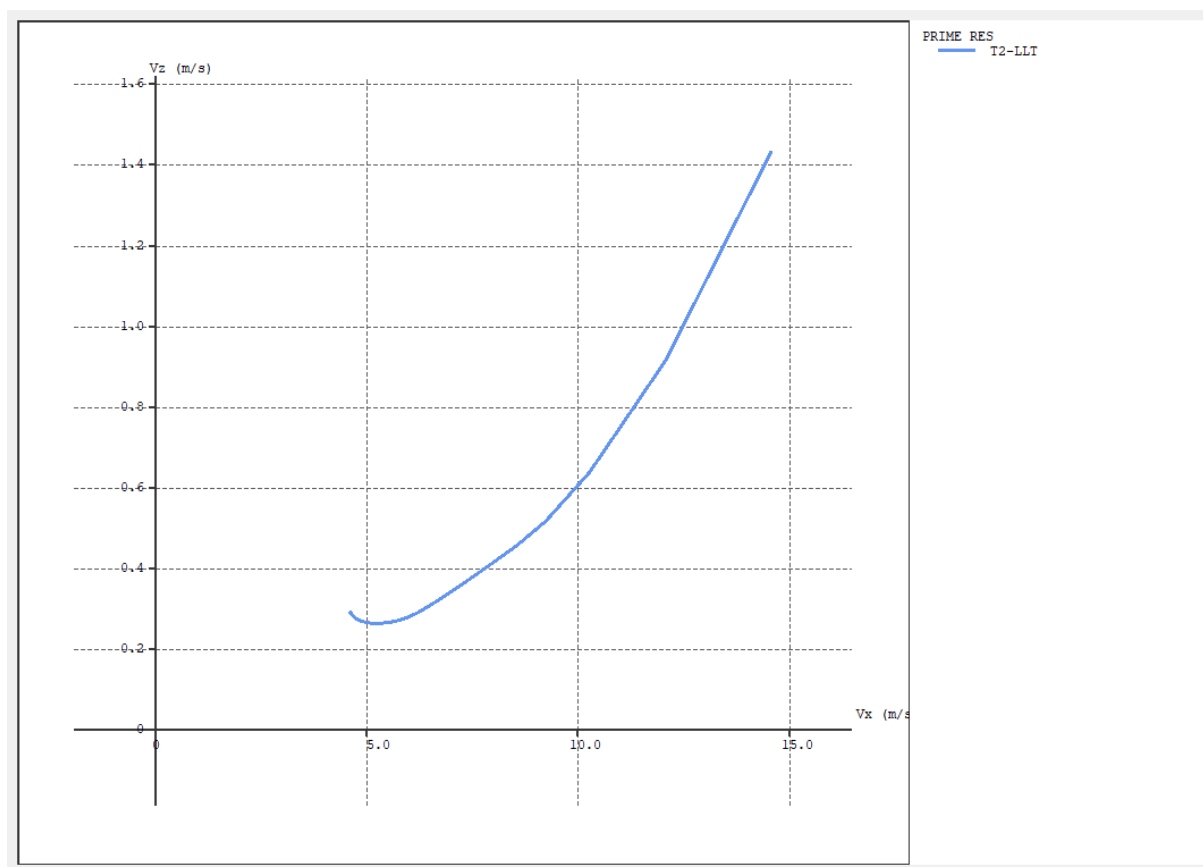
Slika 5.9. Odnos brzine spuštanja i brzine leta jedrilice Prime RES
