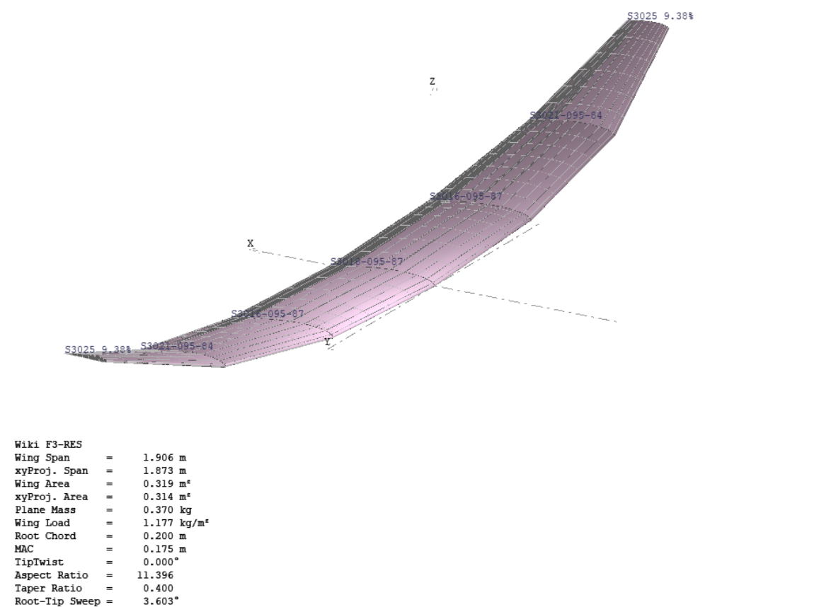
Slika 6.6. Model krila jedrilice Wiki F3L s pripadnim aeroprofilima u programu XFLR5
