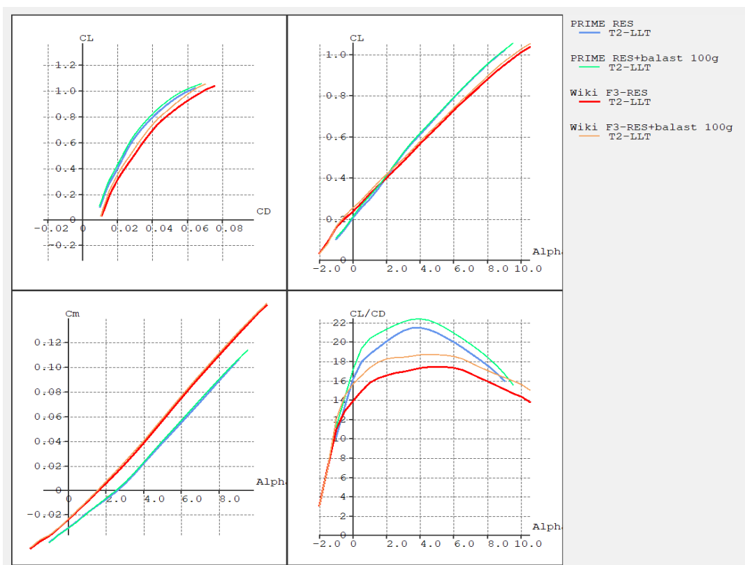
Slika 6.13. Usporedba rezultata analize modela krila originalnog Prime RES i sličnog modela krila Wiki F3L, bez balasta i s dodanim balastom
