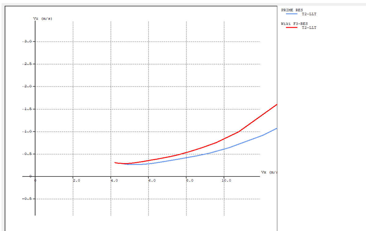
Slika 6.8. Usporedba odnosa brzine spuštavanja i brzine leta jedrilice Prime RES i Wiki F3L
