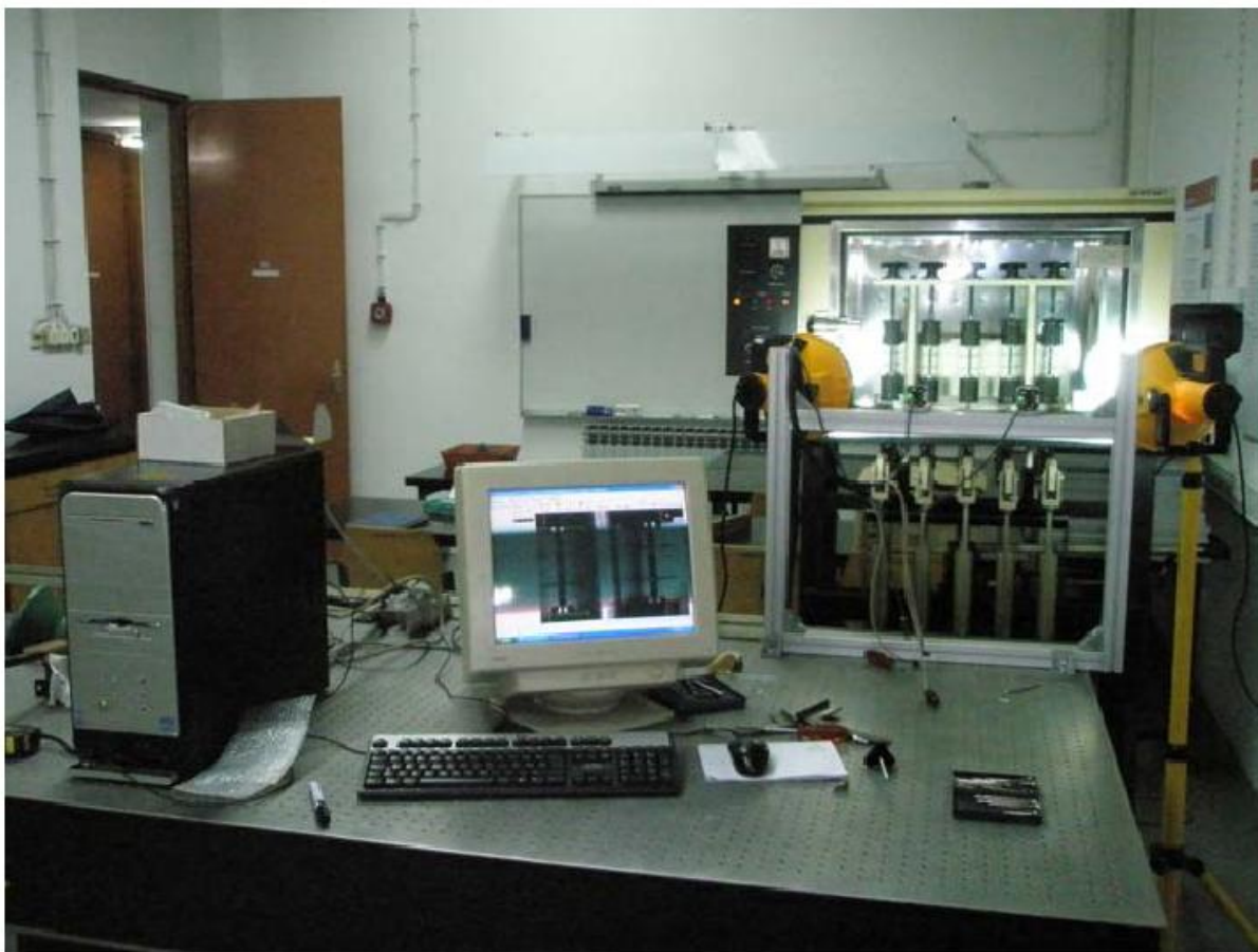
Slika 14 Proces ispitivanja puzanja [3]
