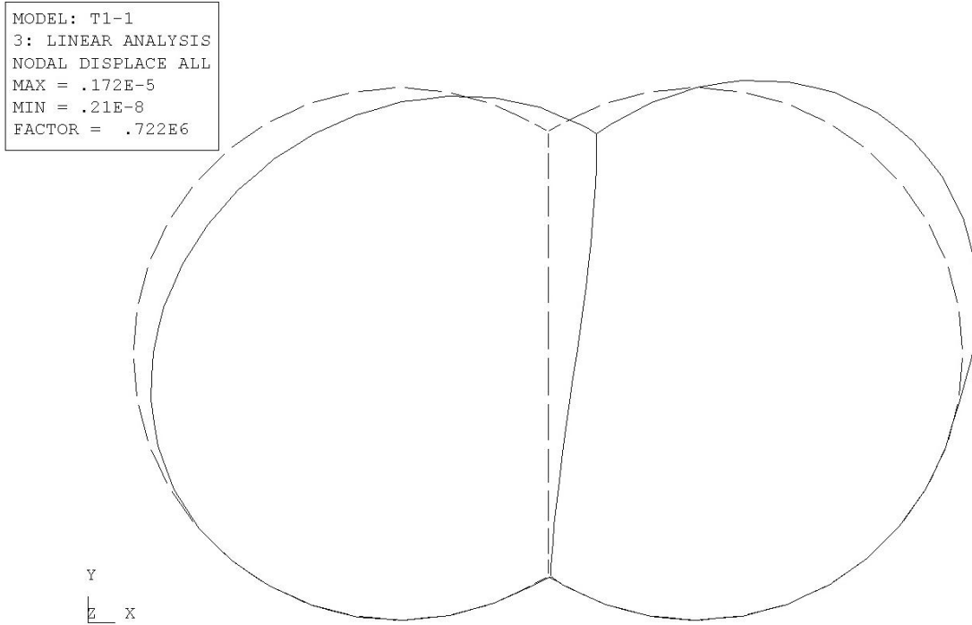
Slika 6.28. Deformacije grednog modela nosivog prstena SR1
