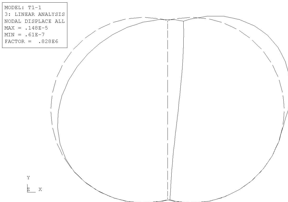
Slika 6.29. Deformacije grednog modela nosivog prstena SR2
