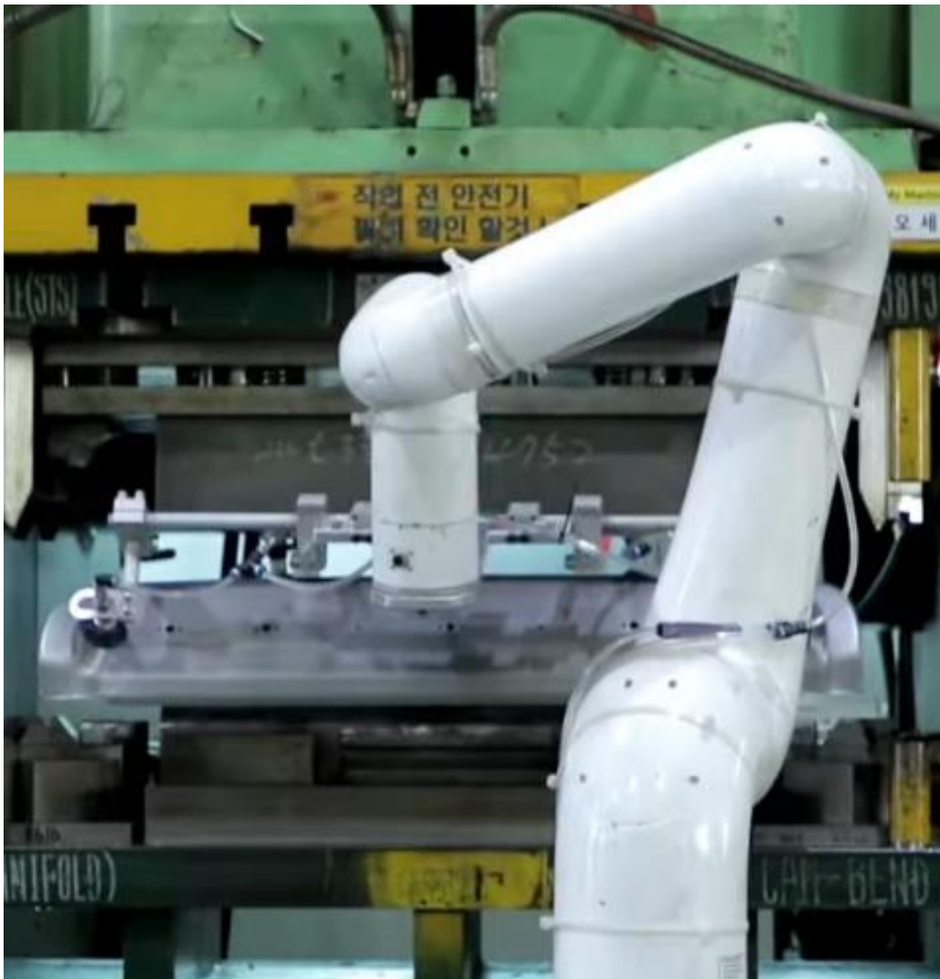
Slika 11. Automatska dostava materijala robotom.[11]
