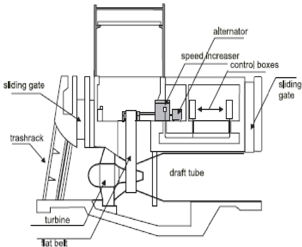
Slika 18. Shema multiplikatora
