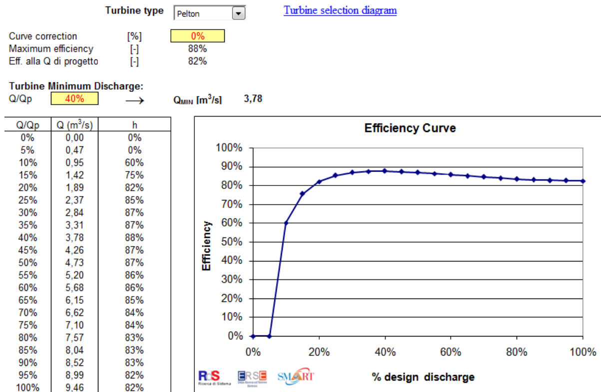
Slika 35. Odabir tipa turbine i prikaz krivulje učinkovitosti turbine
