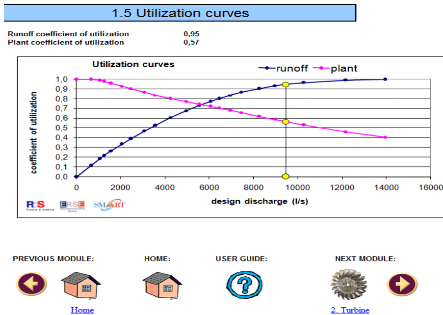
Slika 33. Krivulje iskoristivosti
