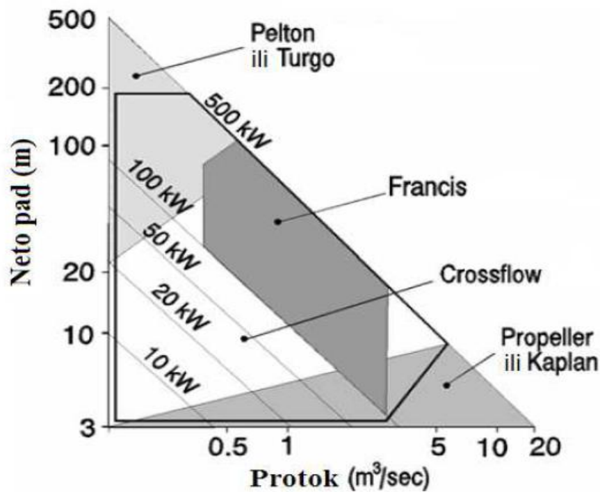
Slika 16. Dijagram područja primjene određenog tipa turbine
