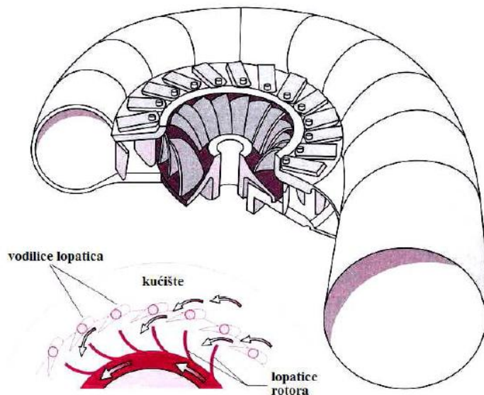
Slika 11. Shema Francis turbine
