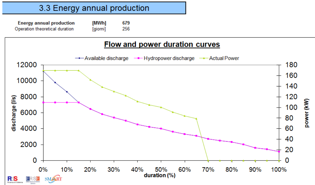
Slika 37. Dijagram trajanja protoka i snage za instalirani protok
