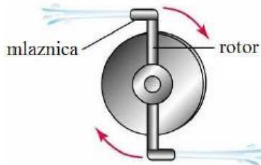
Slika 5. Reakcijska turbina
