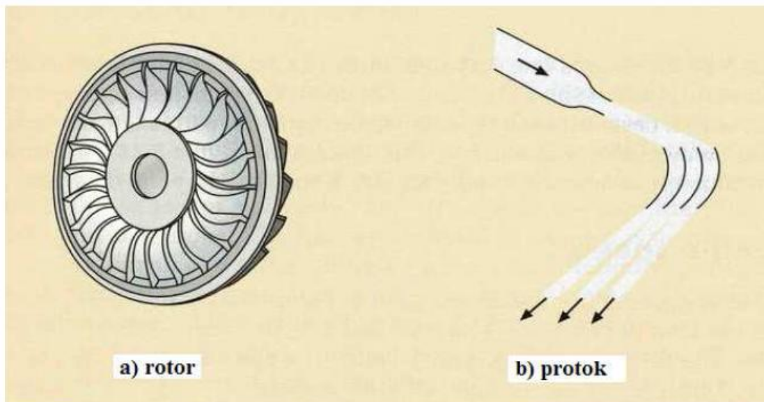
Slika 14. Shema Turgo turbine
