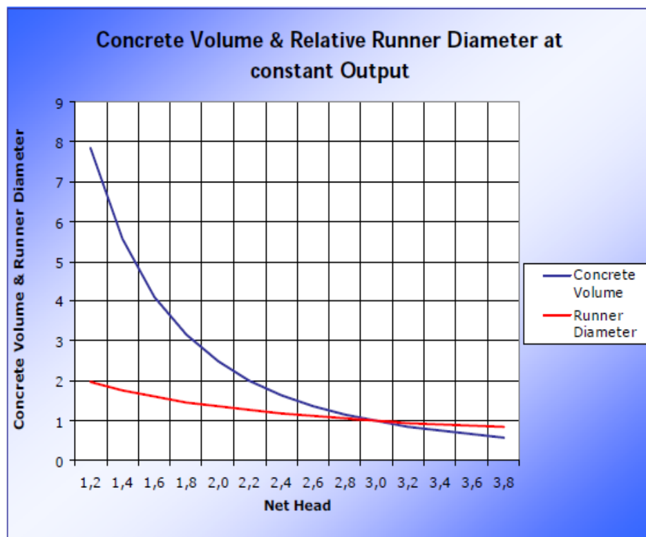
Slika 40. Dijagram povećanja volumena i promjera
