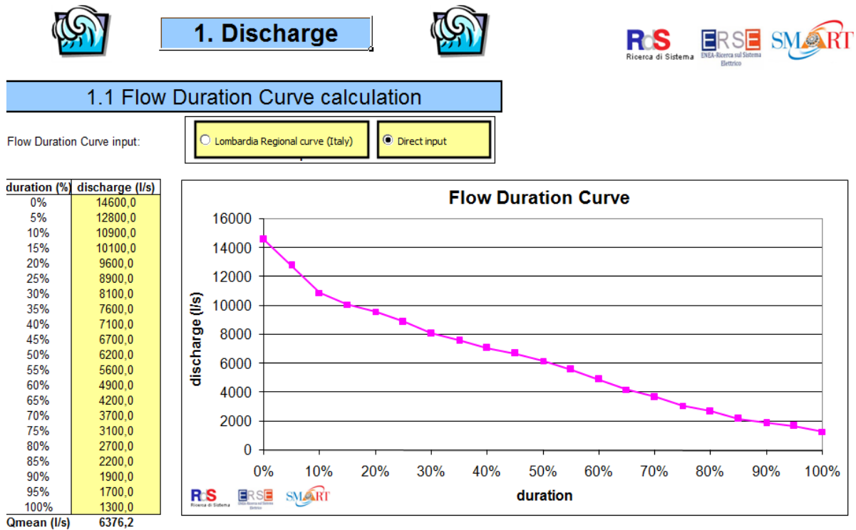
Slika 29. Proračun krivulje trajanja protoka
