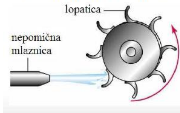
Slika 6. Akcijska turbina
