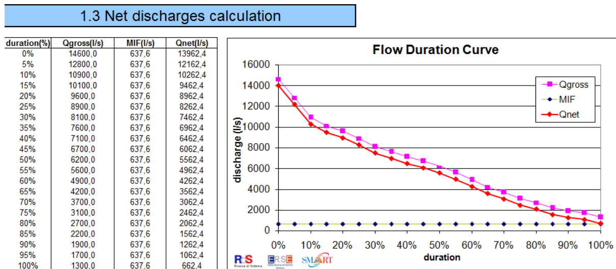
Slika 31. Proračun iskoristivog protoka
