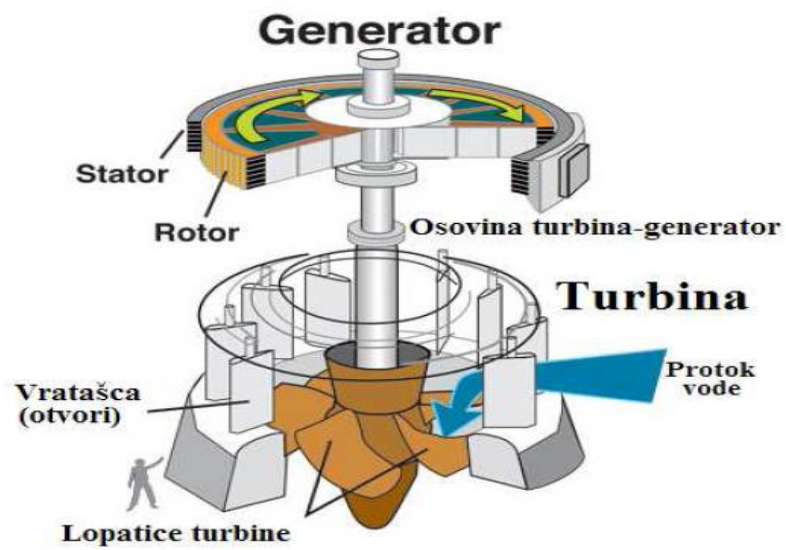
Slika 12. Shema Kaplan turbine
