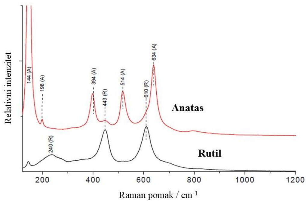
Slika 25 Karakterističan Raman spektar \text{TiO}_2 [124].
