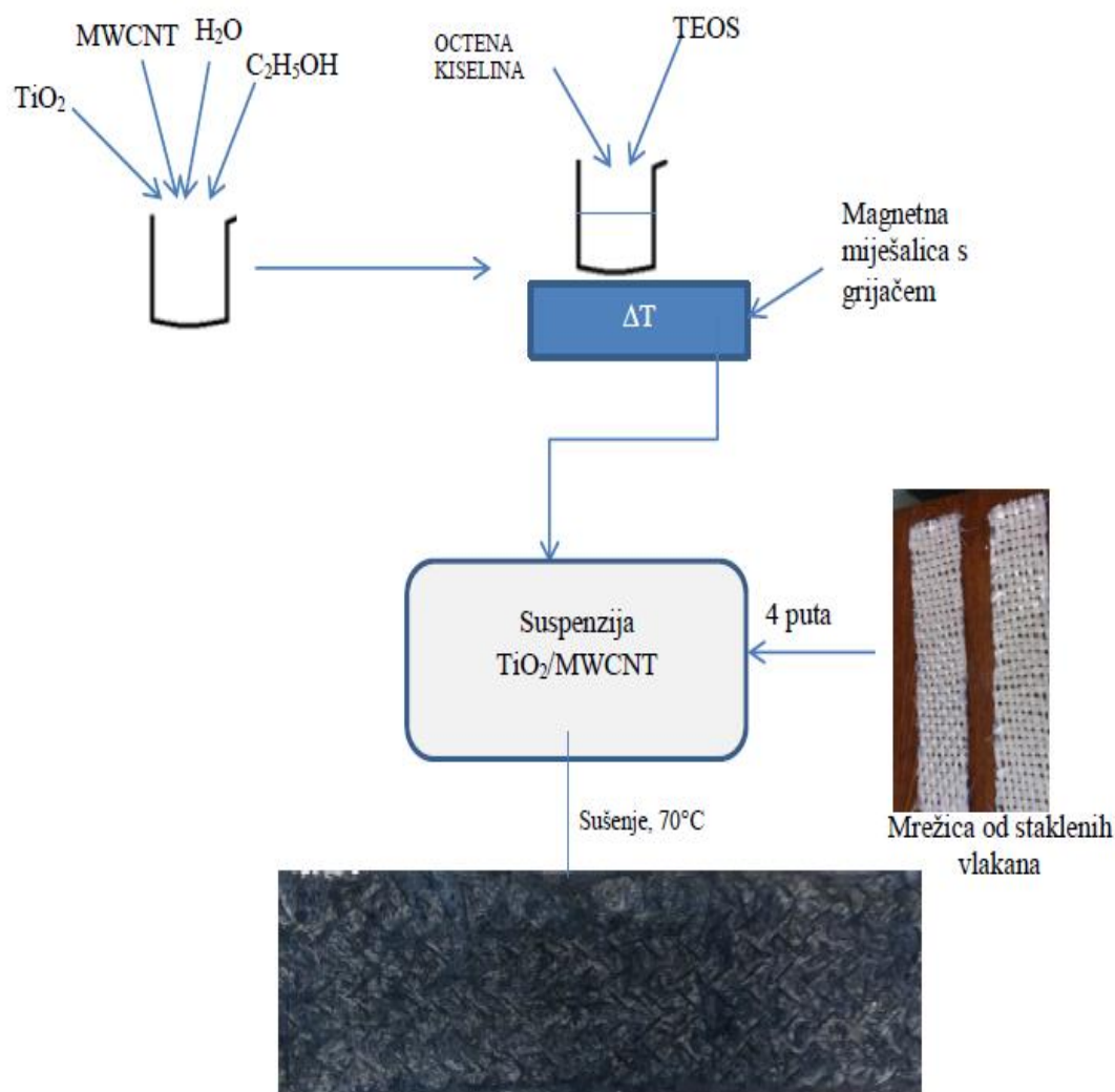
Slika 28 Shematski postupak nanošenja kompozita \text{TiO}_2 / MWCNT na mrežicu od staklenih vlakana.
