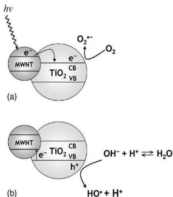
Slika 19 a) MWCNT djeluje kao fotosenzibilator u kompozitu MWCNT / \text{TiO}_2 , b) povratni prijenos elektrona na MWCNT te nastajanje rupe u valentnom pojasu \text{TiO}_2 [94].
