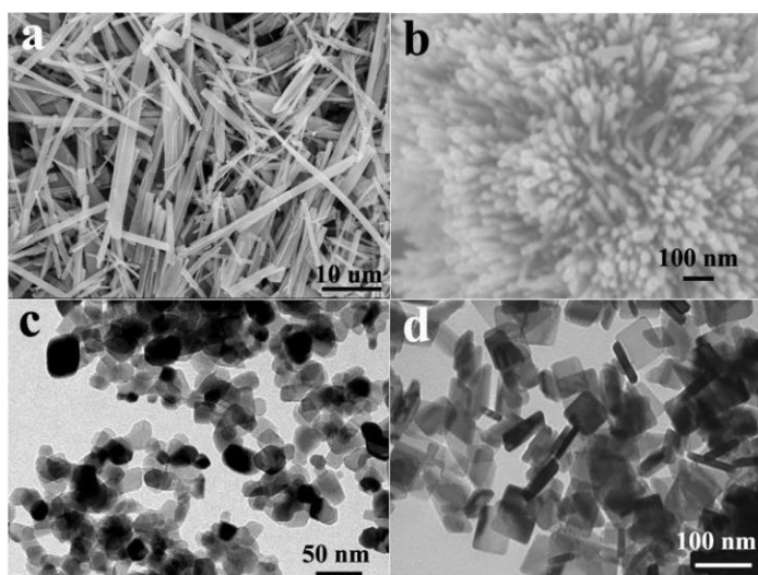
Slika 11 (a) SEM mikrografije \text{TiO}_2 nanoštapica; (b) SEM mikrografije \text{TiO}_2 nanovrpce; (c) TEM mikrografije \text{TiO}_2 Degussa P-25; (d) TEM mikrografije Facettailored-a [31].
