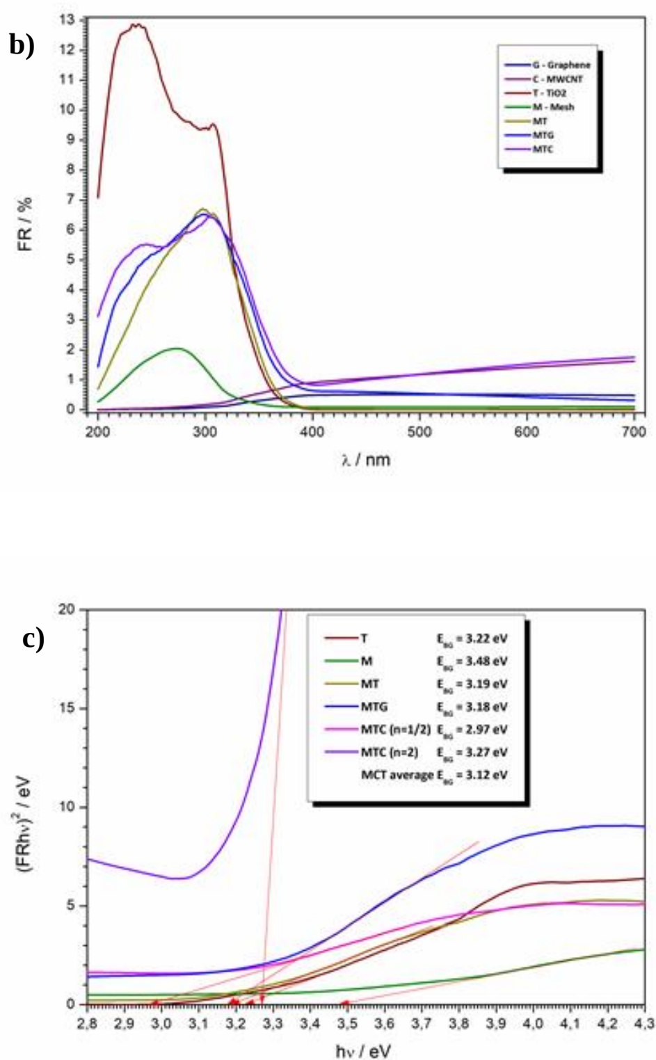
Slika 50 a) DRS UV-Vis spektri, b) Kubelka-Munk spektri refleksije i c) Tauc dijagram za čiste tvari i fotokatalitičke kompozite na staklenoj mreži.
