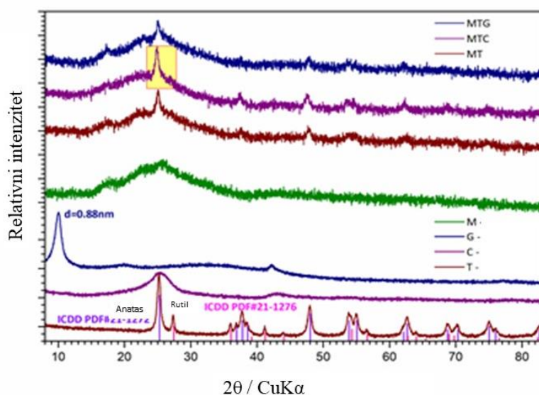
Slika 53 Difraktogrami fotokatalitičkih sastojaka i fotokatalitičkih kompozita na staklenoj mrežici.
