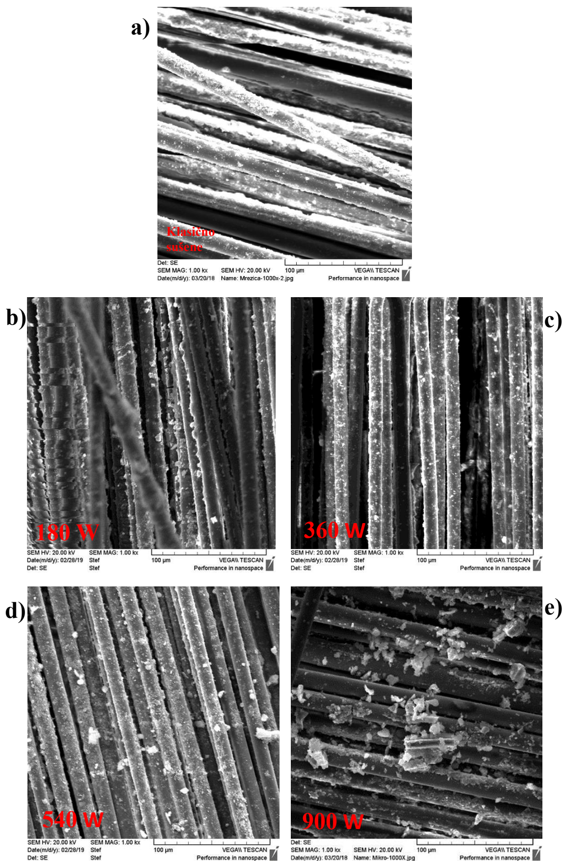
Slika 42 SEM prikaza fotokatalizatora \text{TiO}_2 nanosenog na staklena vlakna i sušenog a) klasično te mikrovalno snagom b) 130 W, c) 360 W, d) 540 W i e) 900 W.
