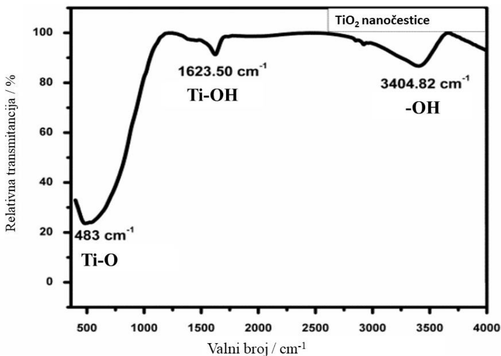
Slika 23 FTIR spektar \text{TiO}_2 [118].
