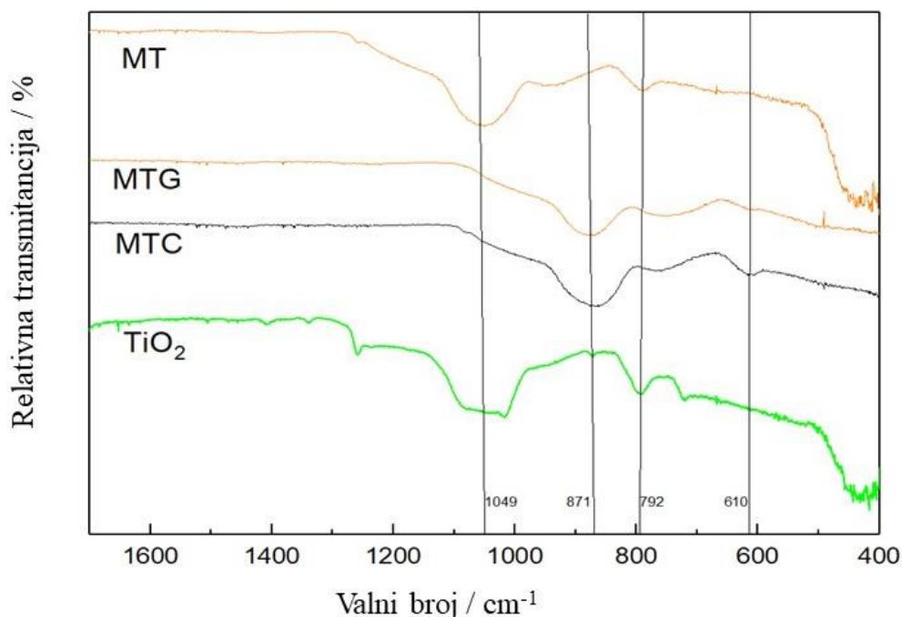
Slika 52 Rezultati FTIR analize imobiliziranih fotokatalizatora na staklenu mrežicu sa karakterističnim vrhovima.
