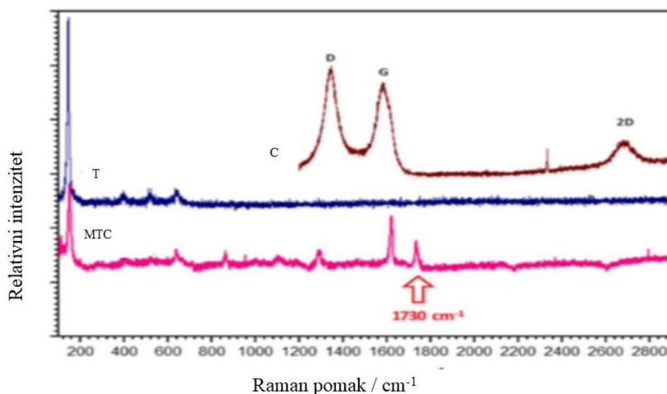
Slika 54 Raman spektri fotokatalitičkih sastojaka i fotokatalitičkih kompozita na staklenoj mrežici [137].
