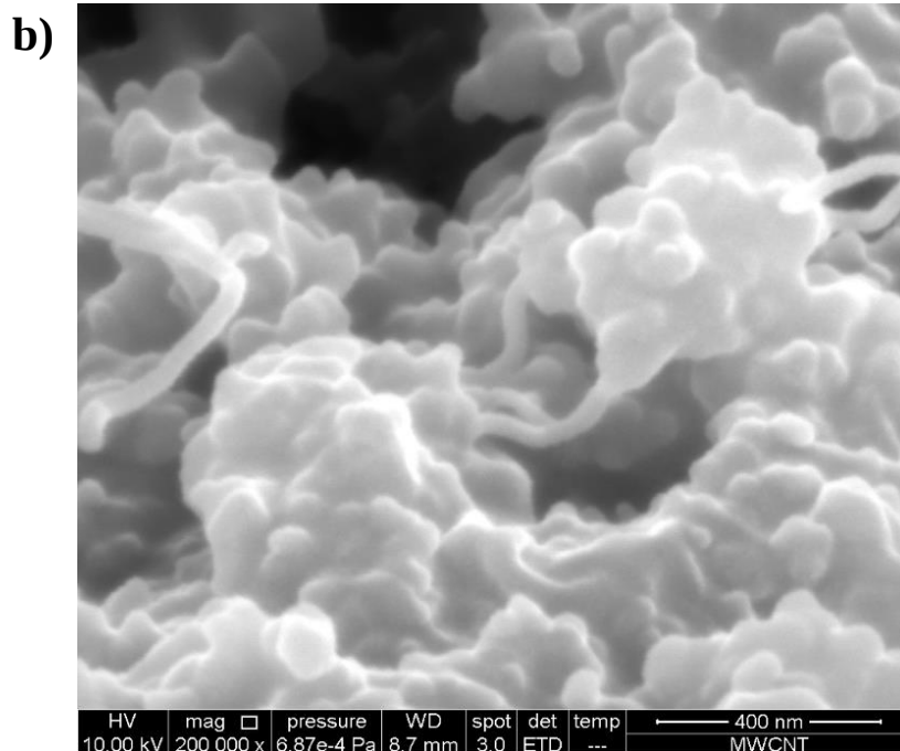
Slika 55 Imobilizirani slojevi TiO 2 i MWCNT pri povećanju od a) 1000 x i b) 200 000 x.
