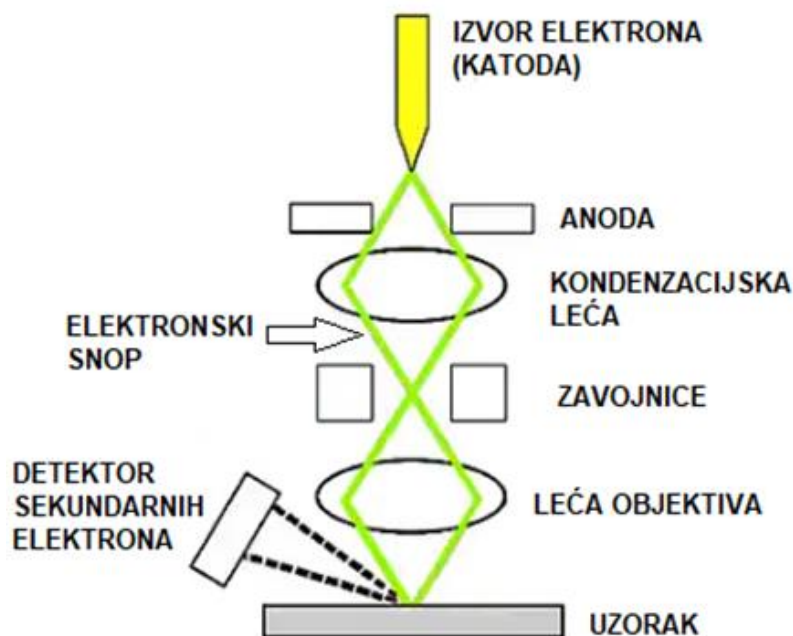
Slika 22 Shematski prikaz principa rada pretražnog elektronskog mikroskopa [110].
