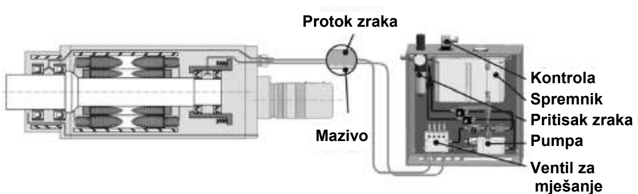
Slika 4.7. Prikaz sustava podmazivanja ulje - zrak za motorvretena [2]
