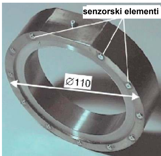
Slika 6.4. Mjerni prsten s piezoelektričnim senzorima sile [2]
