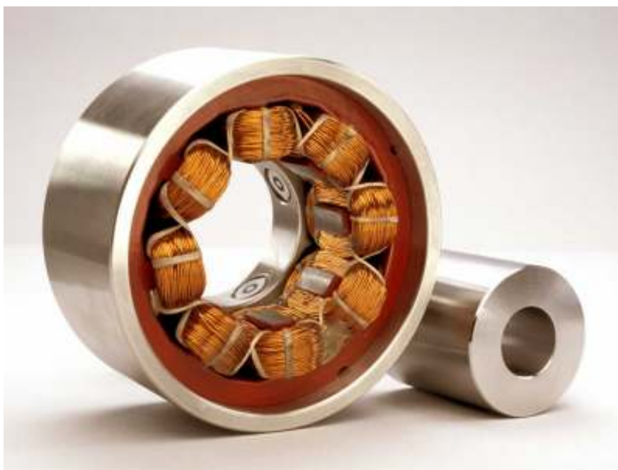
Slika 4.6. Magnetski ležaj [5]
