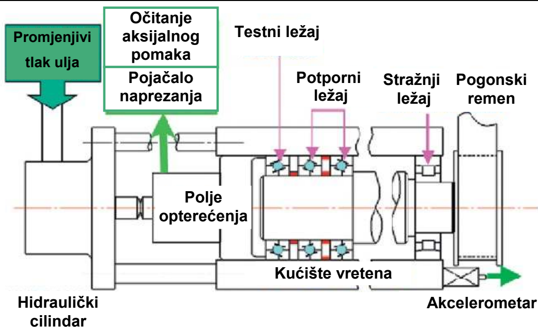
Slika 6.3. Shema ispitnog uređaja ležajeva [2]
