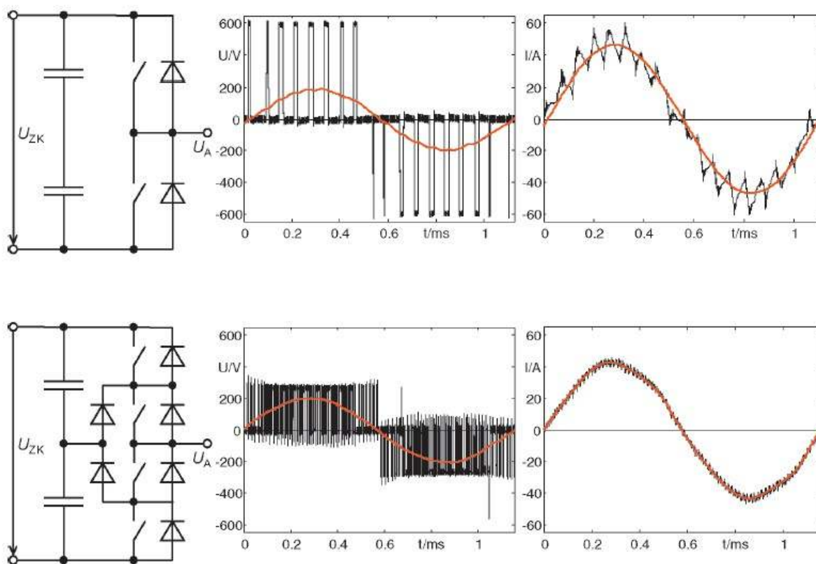
Slika 5.2. Shema, naponi i struje dvorazinskog(gore) i torazinskog(dolje) pretvarača [2]
