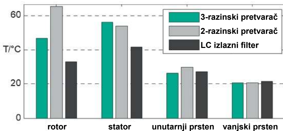
Slika 5.3. Stacionarne temperature motora i prednjeg ležaja s tri različita pretvarača frekvencije [2]
