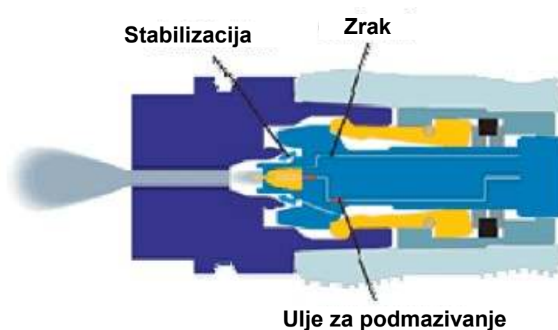
Slika 4.12. Izbjegavanje razdvajanja aerosola [7]
