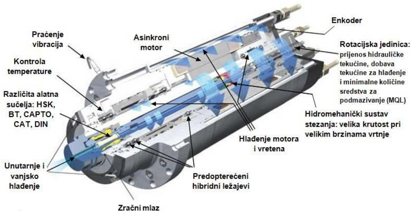
Slika 2.2. Presjek motorvretena [3]
