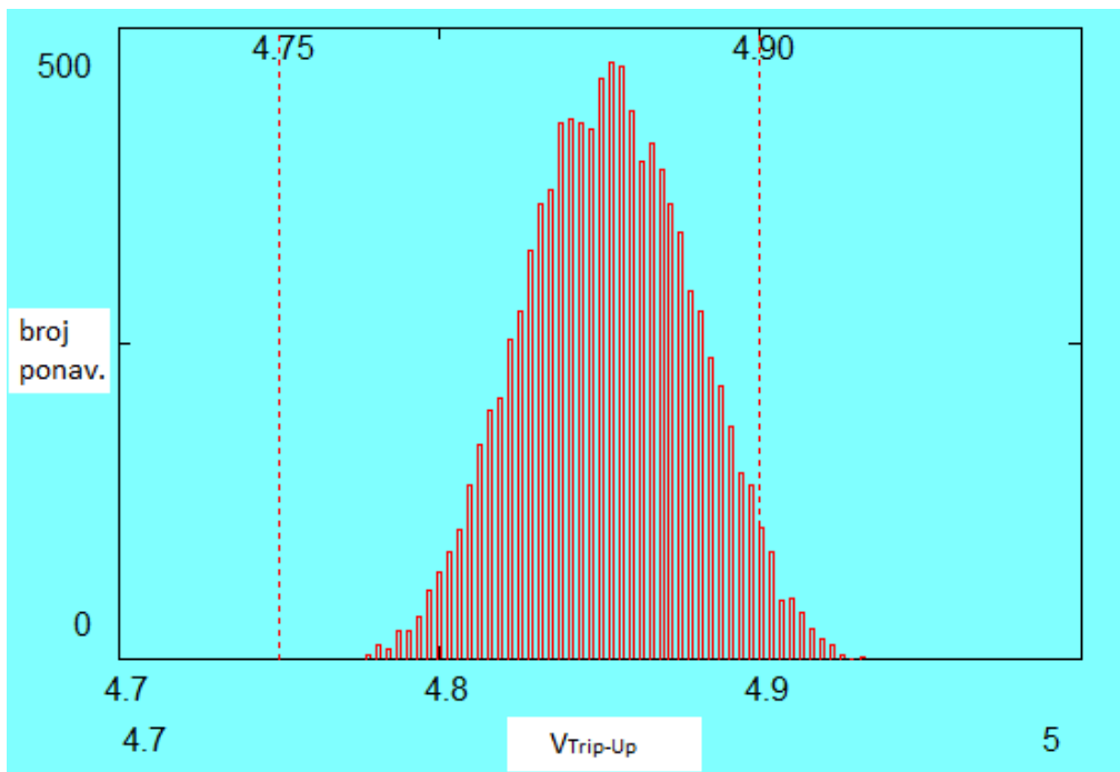
Slika 7. Dijagram funkcije rasipanja za V_{trip-up} generirana u Mathcad-u
