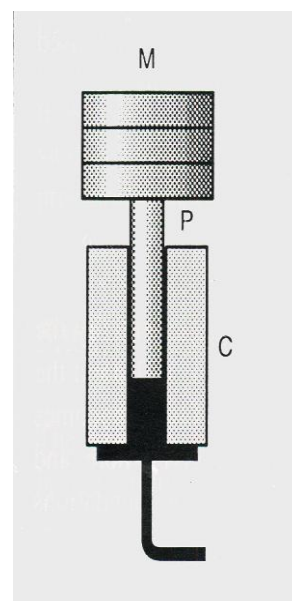
Slika 6. Tlačna vaga korištena prilikom laboratorijskog umjeravanja
