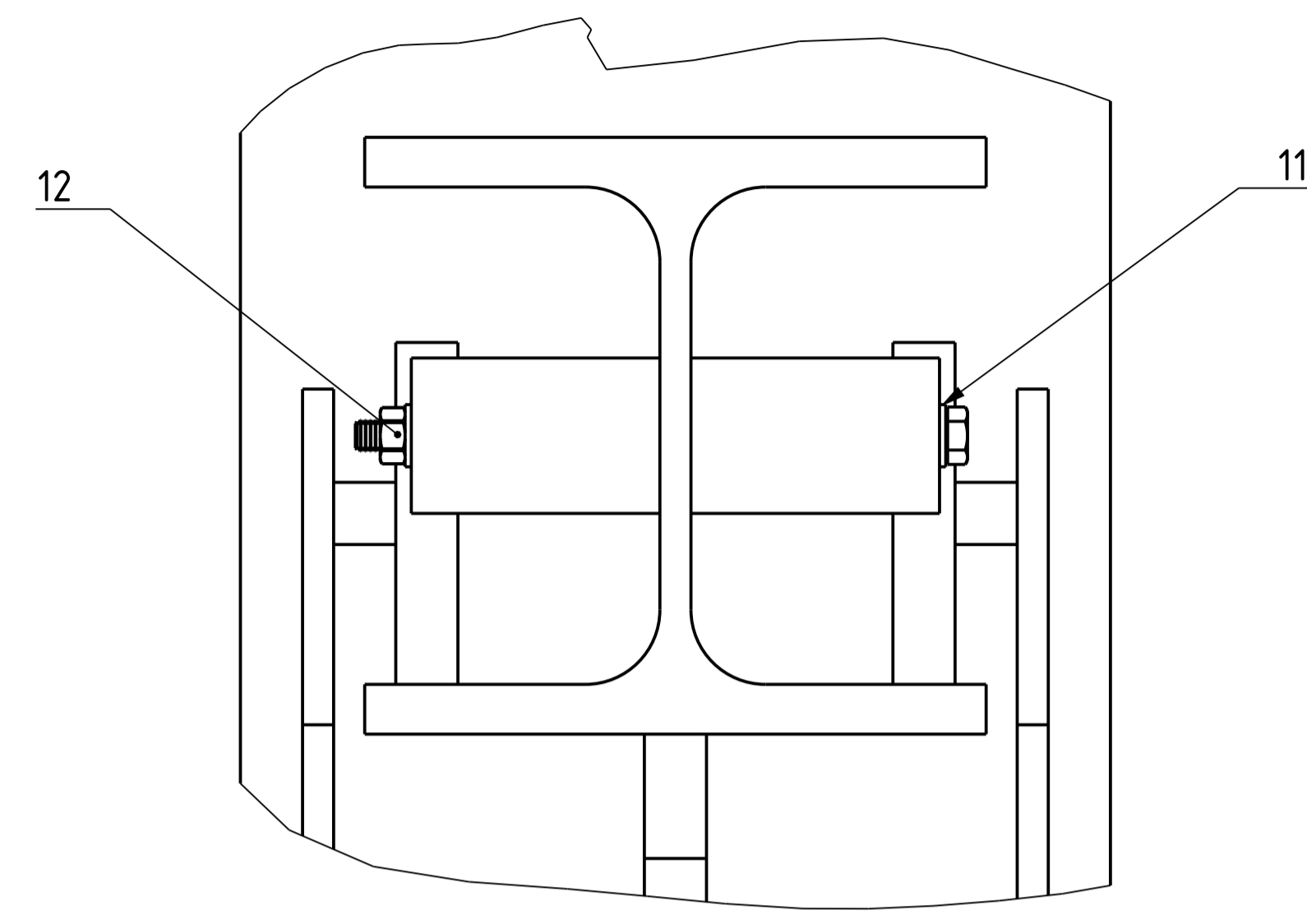
B Mjerilo 1:5
