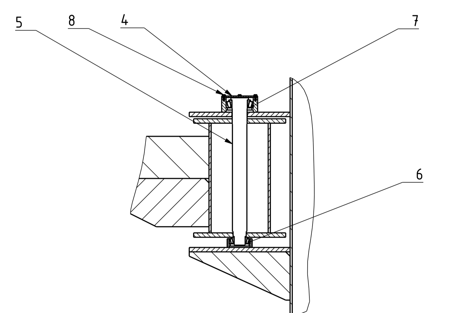
B Mjerilo 1:5
