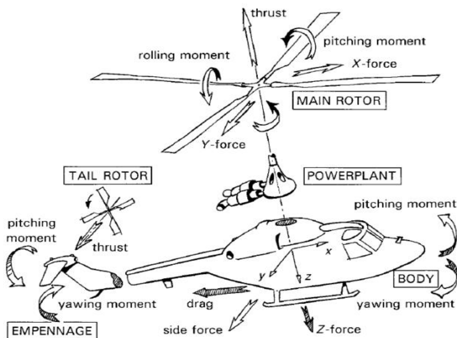
Slika 3.1 Sile i momenti koji djeluju na helikopter [2]
