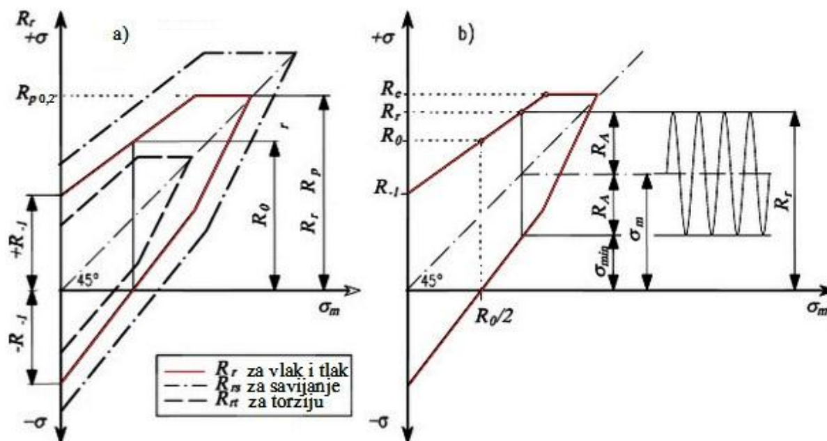
Slika 41. Smithov dijagram trajne dinamičke čvrstoće: a) za različite vrste opterećenja, b) Smithov dijagram za poznate tri karakteristike čvrstoće R_1 , R_0 , R_r
