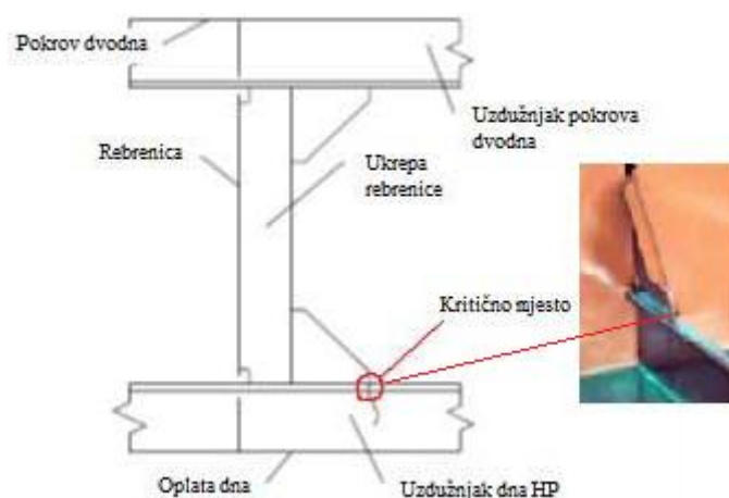
Slika 12. Kritično mjesto pojave zamornog oštećenja - dvodno tankera [5]
