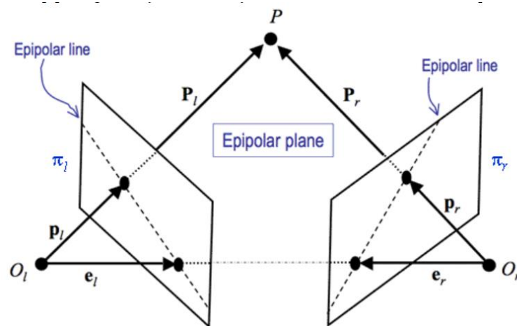
Slika 4. Prikaz epipolarnog ograničenja [9]
