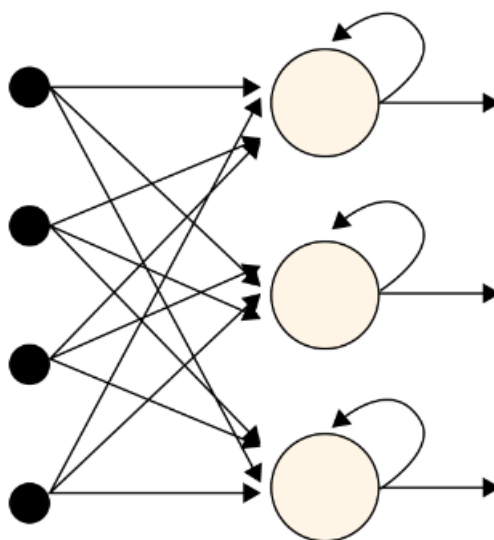
Slika 13. Rekurentna neuronska mreža [18]
