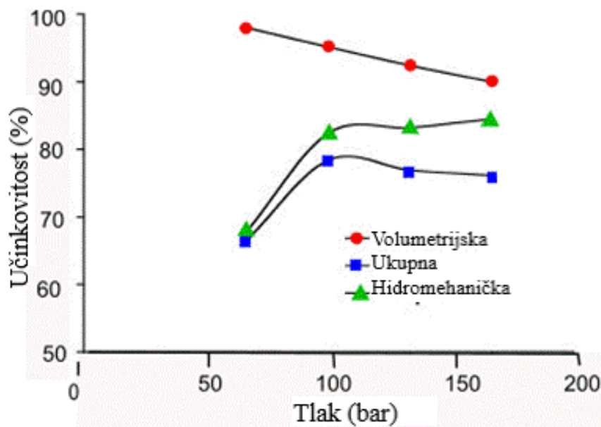
Slika 5. Karakteristike zupčanih hidraulički pumpe [9]
