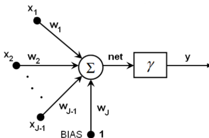
Slika 10. Model statički neuron [14]
