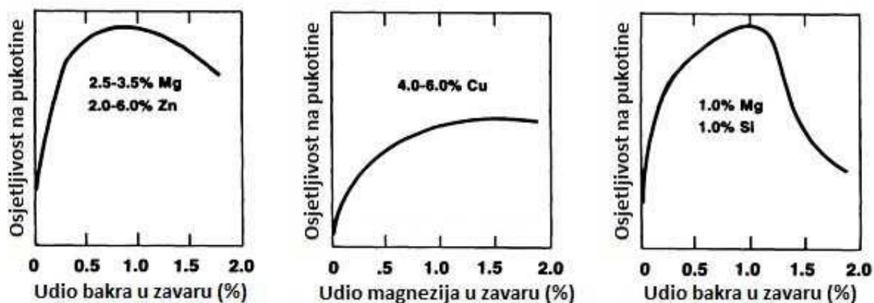
Slika 32. Osjetljivost na stvaranje pukotina aluminijskih legura sa više legirnih elemenata [27]
