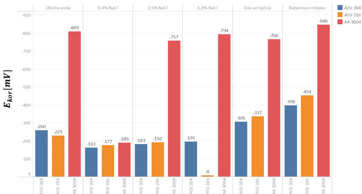
Slika 33. Graf odnosa rezultata korozivnog potencijala različitih uzoraka za različiti elektrolit
