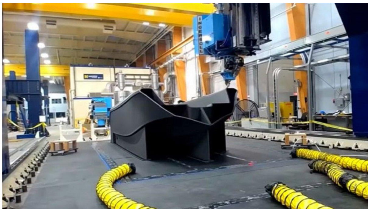
Slika 16. 3D ispisan trup plovila [21]
