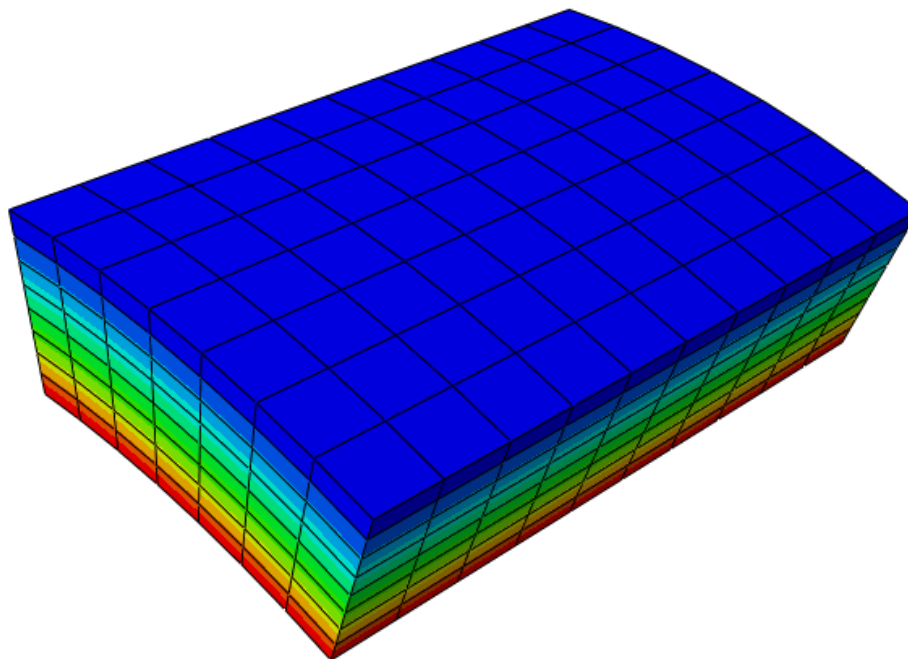
Slika 14. Raspodjela cirkularnog naprezanja za NH
