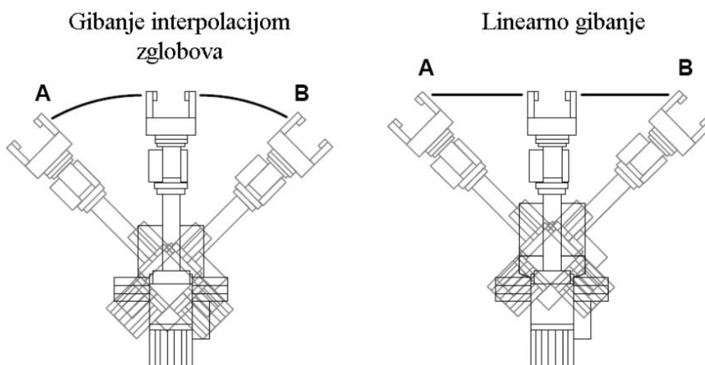
Slika 33. Prikaz vrste gibanja robota [23]
