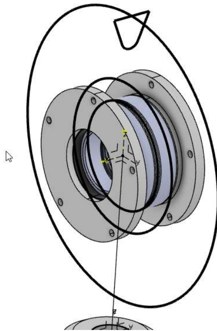
Slika 46. Kostur geometrija užnice
