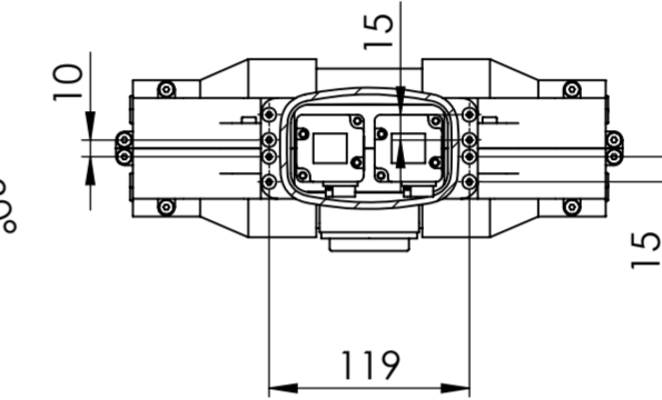
PRESJEK F-F MJERILO 2:1
