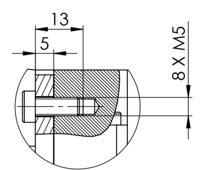
DETALJ E MJERILO 1:1
