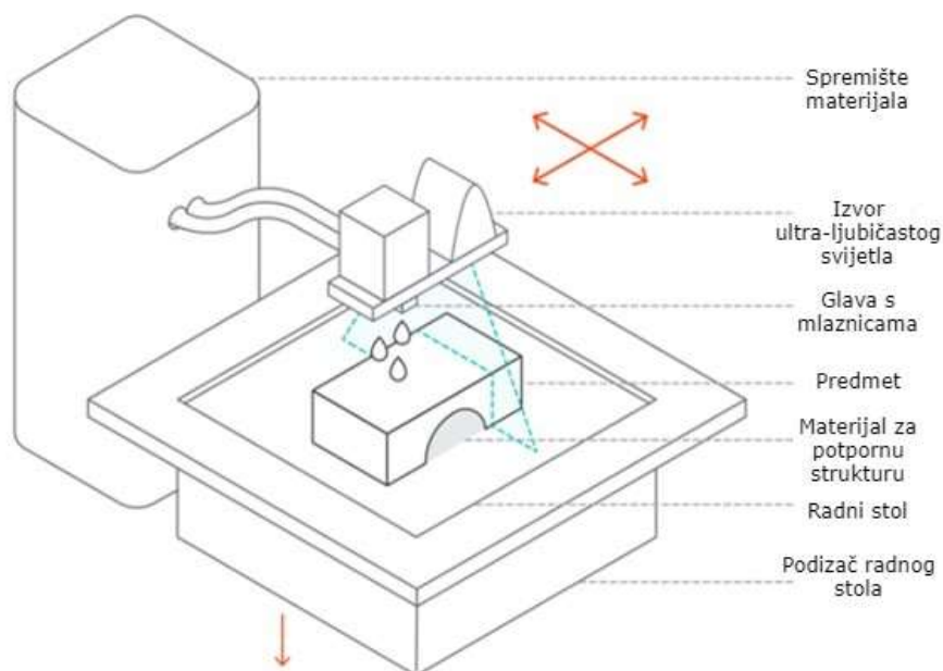
Slika 6. PolyJet postupak [13]
