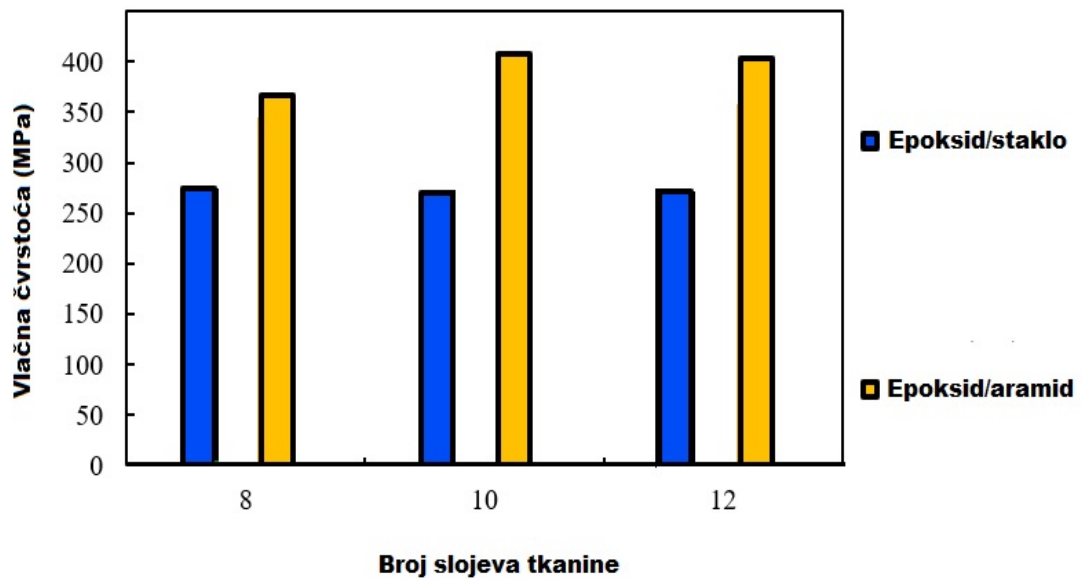
Slika 18. Literaturne vrijednosti vlačne čvrstoće kompozitnih materijala [59]
