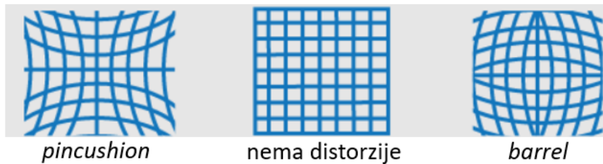
Slika 2.6. Vrste radijalne distorzije [10]
