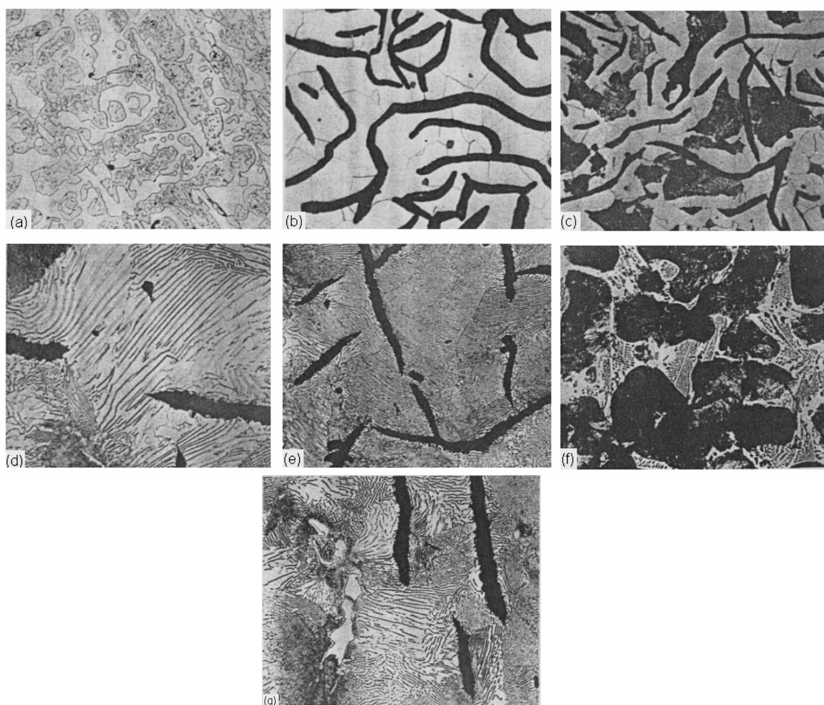
Slika 13. Struktura željeznih ljevova (a) Bijeli ljev (perlit + \text{Fe}_3\text{C} ), H_B 550. (b) Sivi ljev (listići grafita u feritnoj željeznoj osnovi), H_B 120. (c) Sivi ljev (grafit u feritnoj-perlitnoj željeznoj osnovi), H_B 150. (d) Sivi ljev (grafit u gruboj perlitnoj željeznoj osnovi), H_B 195. (e) Sivi ljev (grafit u finoj perlitnoj željeznoj osnovi), H_B 215. (f) Sivi ljev (grafit u perlitnoj-steaditnoj željeznoj osnovi), H_B 200. (g) Sivi ljev (grafit u perlitnoj- karbidnoj osnovi), H_B 240.
