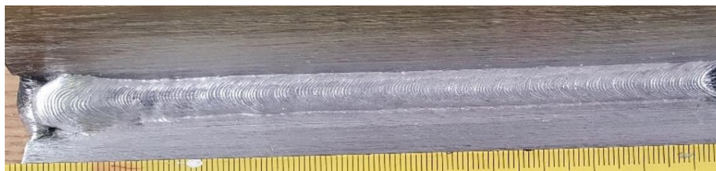
Slika 45. Naličje kutnog zavara A2 izvedenog u zaštiti 100% argona uz f=20 Hz
