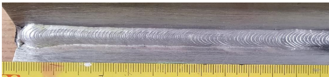
Slika 43. Naličje kutnog zavara A1 izvedenog u zaštiti 100% argona uz f=8 Hz
