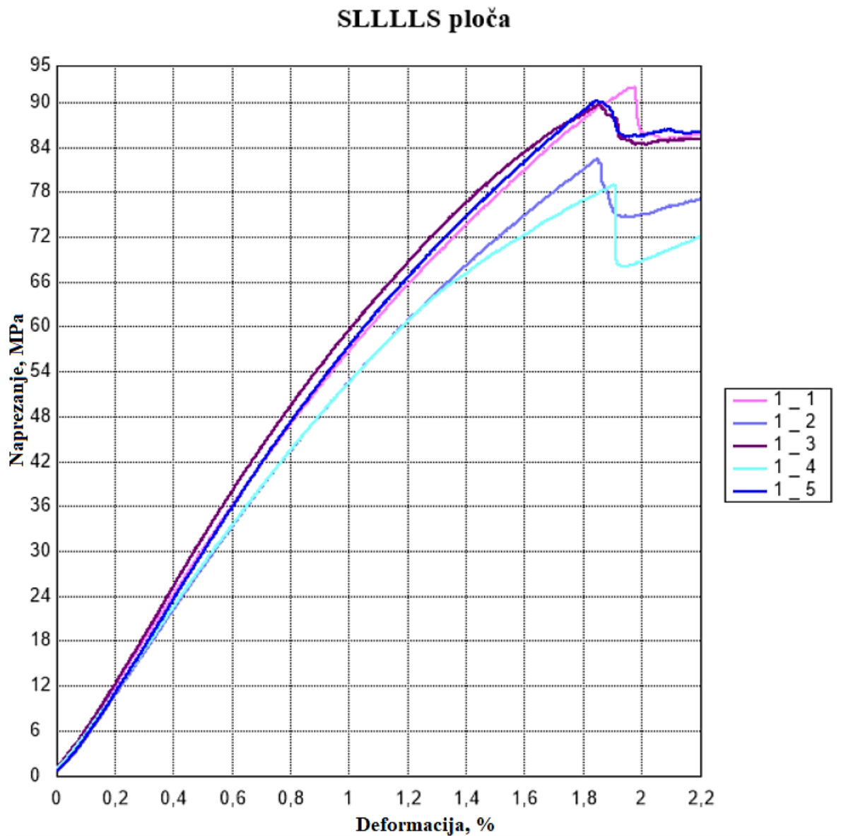
Slika 32. Dijagrami savojno naprezanje-istezanje za SLLLLS ploču
