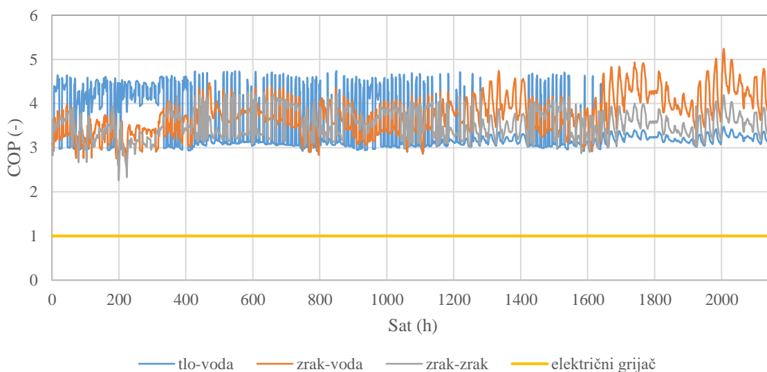
Slika 31 Učinkovitost sustava u režimu grijanja u prvom tromjesečju
