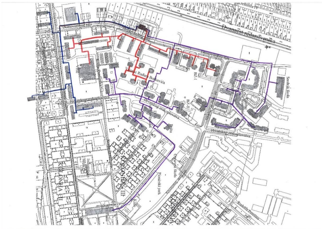
Slika 7 Distribucijska mreža - CTS Borovo naselje
