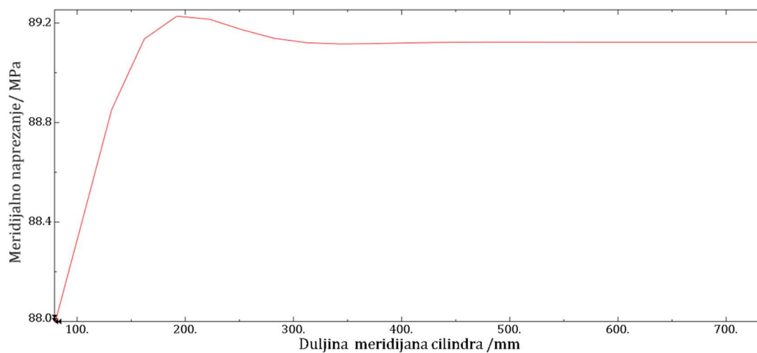
Slika 75. Raspodjela meridijalnog napreznja duž meridijana cilindra
