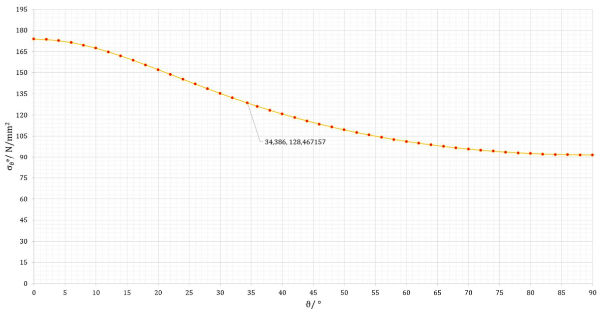
Slika 23. Raspodjela meridijalnog naprezanja u ovisnosti kuta \vartheta
