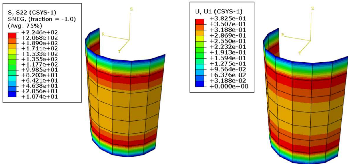
Slika 52. Prikaz rezultata cirkularnog napreznja (lijevo) i radijalnog pomaka (desno) za generiranu mrežu od 56 S4 elemenata
