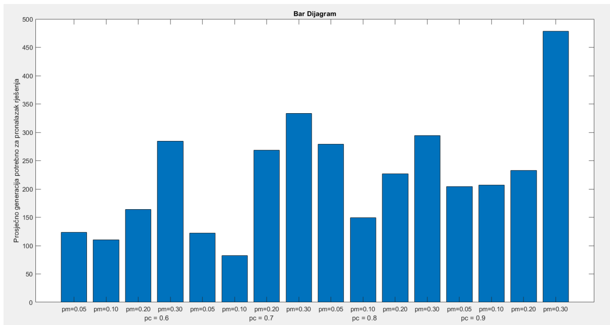
Slika 5 Histogram 2
