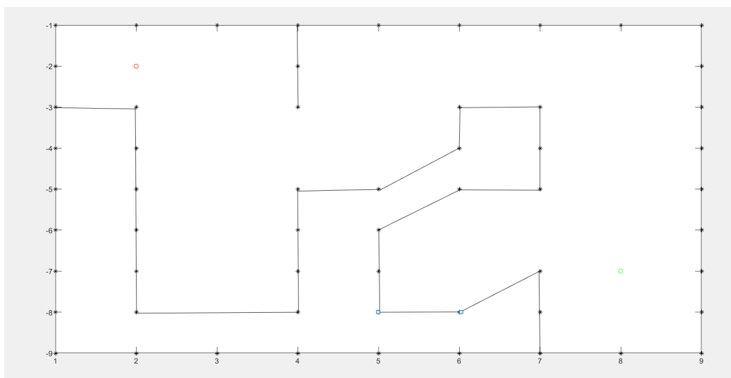
Slika 18 Drugi labirint
