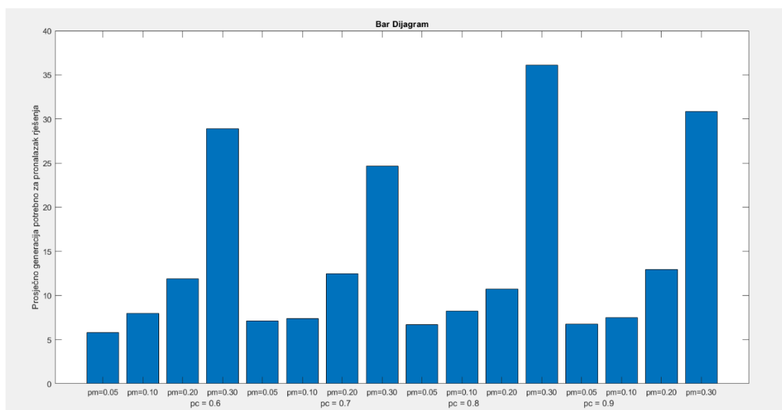
Slika 7 Histogram 3
