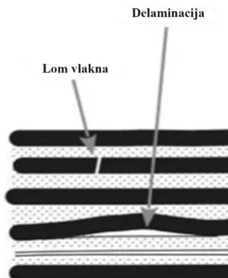
Slika 9. Delaminacija [6]
