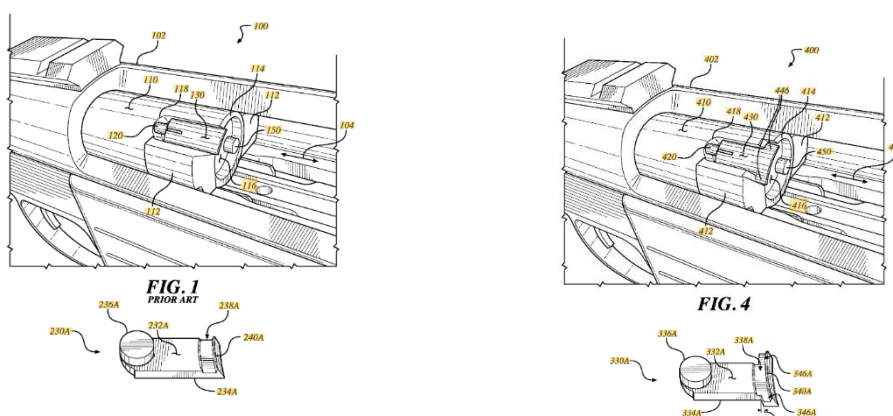
Slika 41. Usporedba Sako izvlačača i izvlačača produženog zaglavlja
