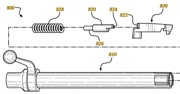
Slika 42. Sklop izvlačača
