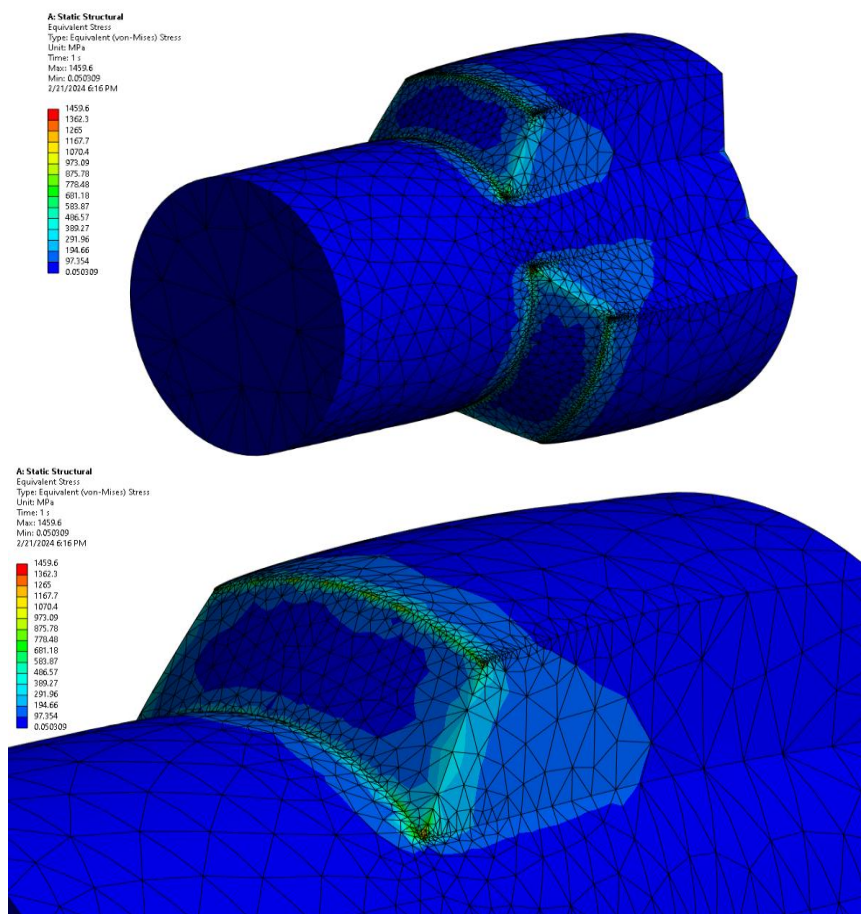
Slika 74. Prikaz rezultata usitnjene mreže - naprezanja
