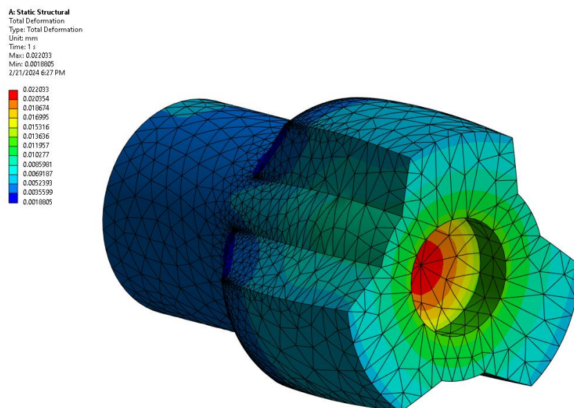
Slika 75. Prikaz rezultata statičke analize usitnjene mreže - deformacija
