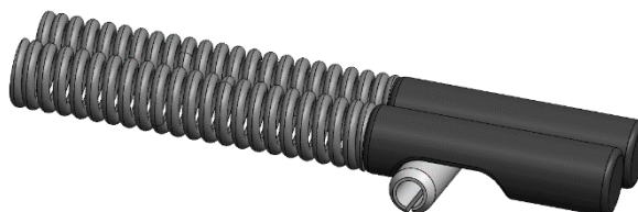
Slika 56. Sklop izbacivača
