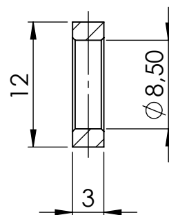
A-A (M 2:1)
