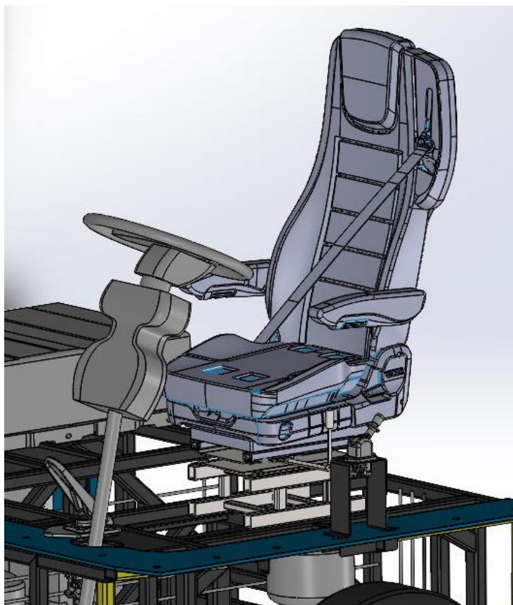
Slika 25. Sklop mehanizma pričvršćen na cijevi šasijske – prostorni prikaz
