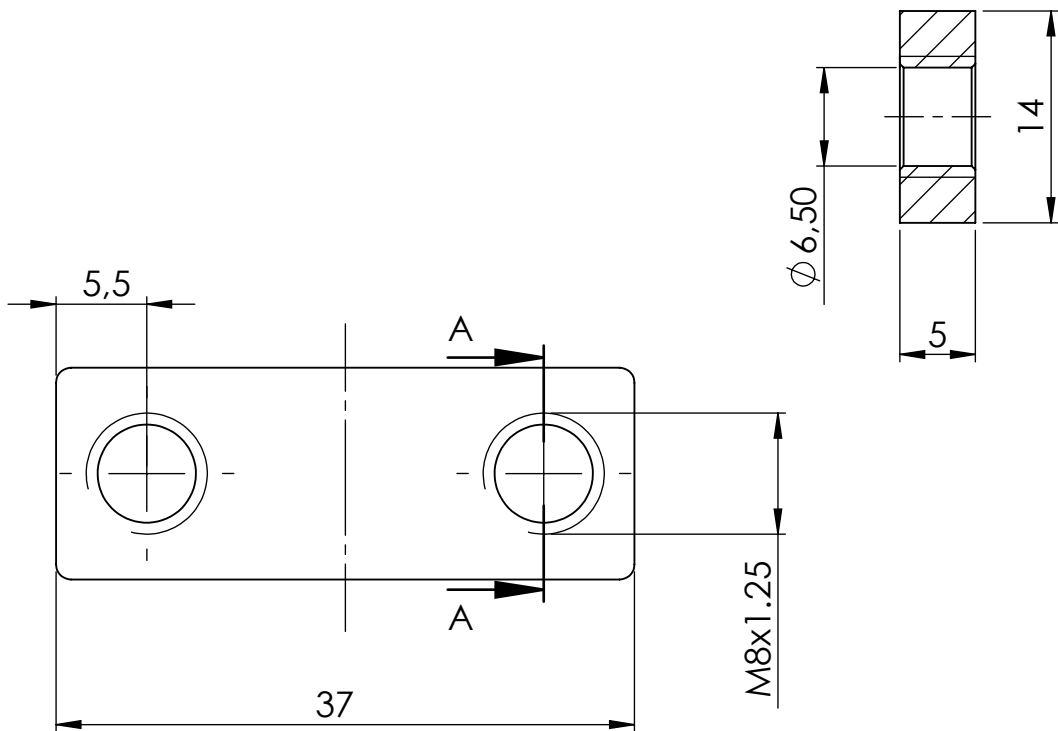
A-A (M 2:1)
