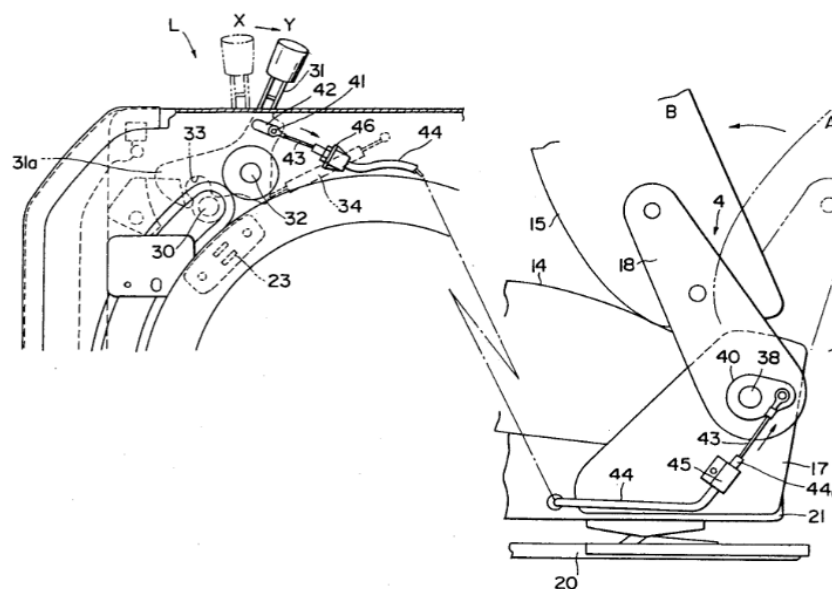
Slika 12. Nagnuto sjedalo [11]
