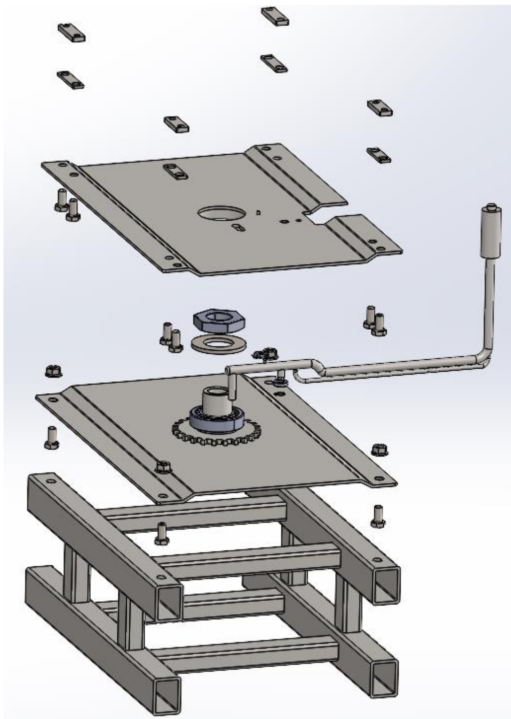
Slika 22. Prikaz svih komponenti mehanizma
