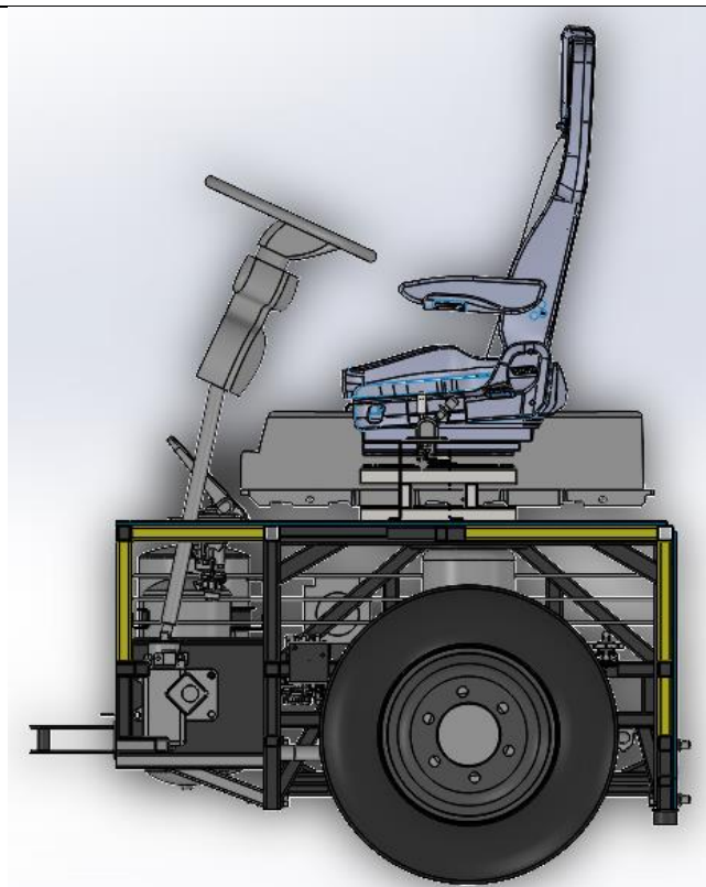
Slika 24. Sklop mehanizma pričvršćen na cijevi šasijske – pogled s boka
