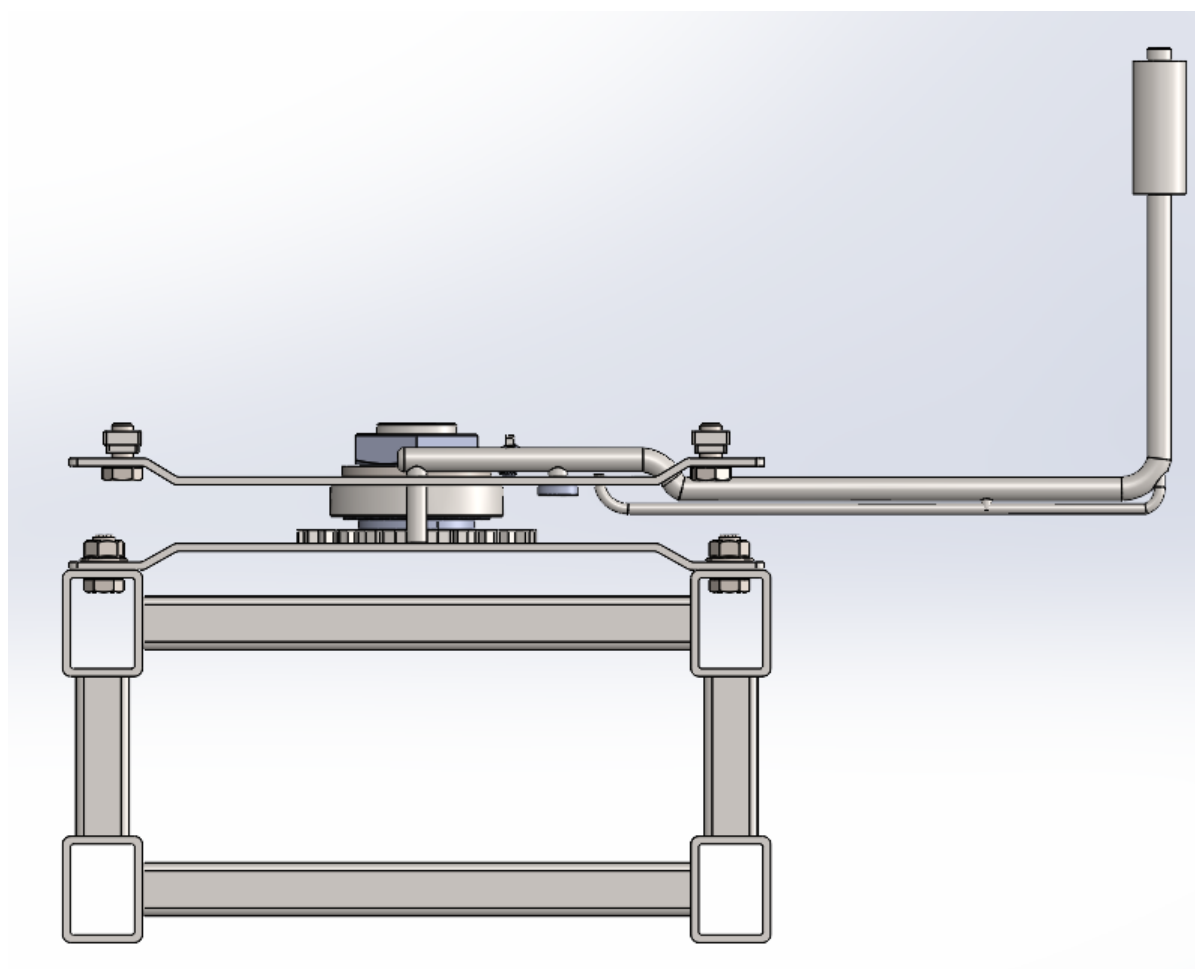
Slika 21. Mehanizam zakretanja
