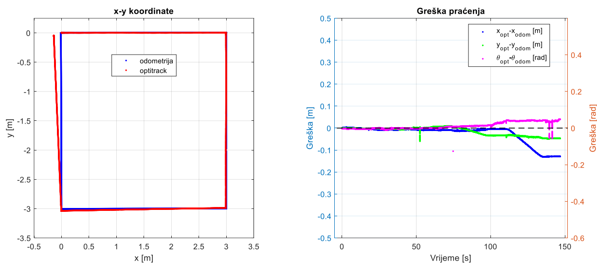
Slika 42. 5. mjerenje nakon implementacije kalibracije UMBmark metode u smjeru kazaljke na satu
